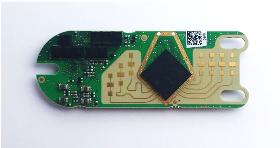
880870_Slave_Radar-Board_BOTTOM
