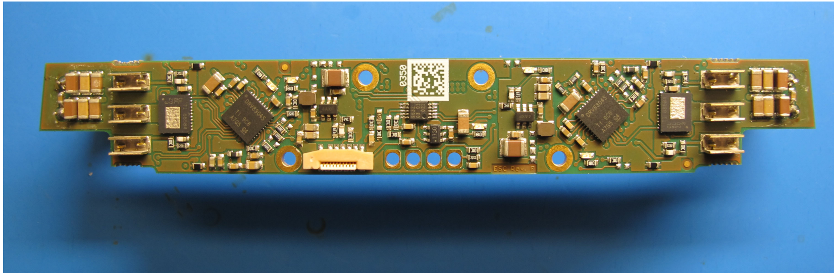
891019_ESC-Board_BOTTOM
