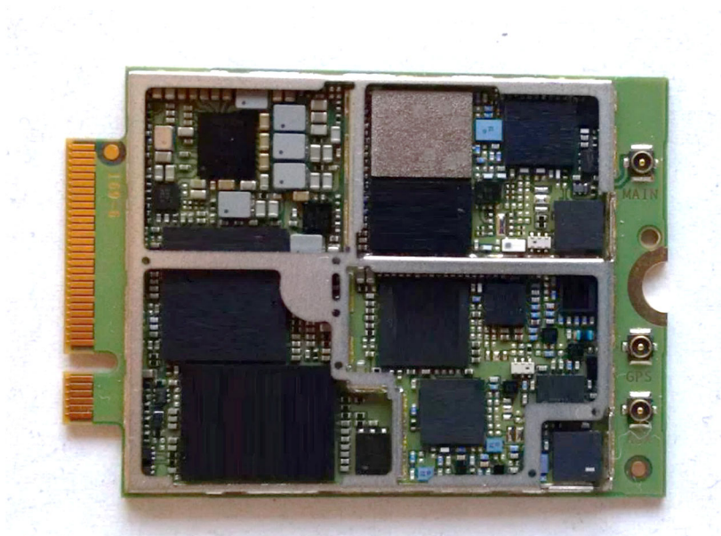
897756_LTE Bottom
