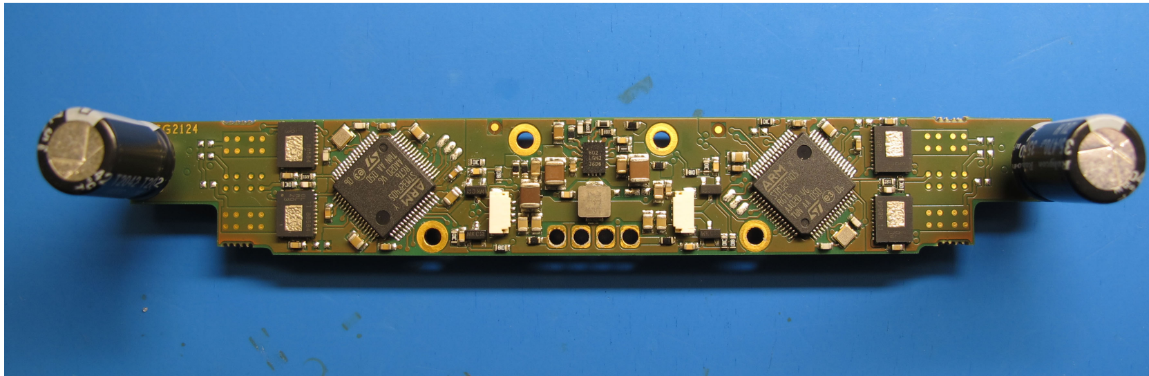
891019_ESC-Board_BOTTOM
