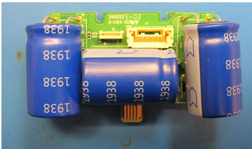
881218_Supercap-Board-BOTTOM
