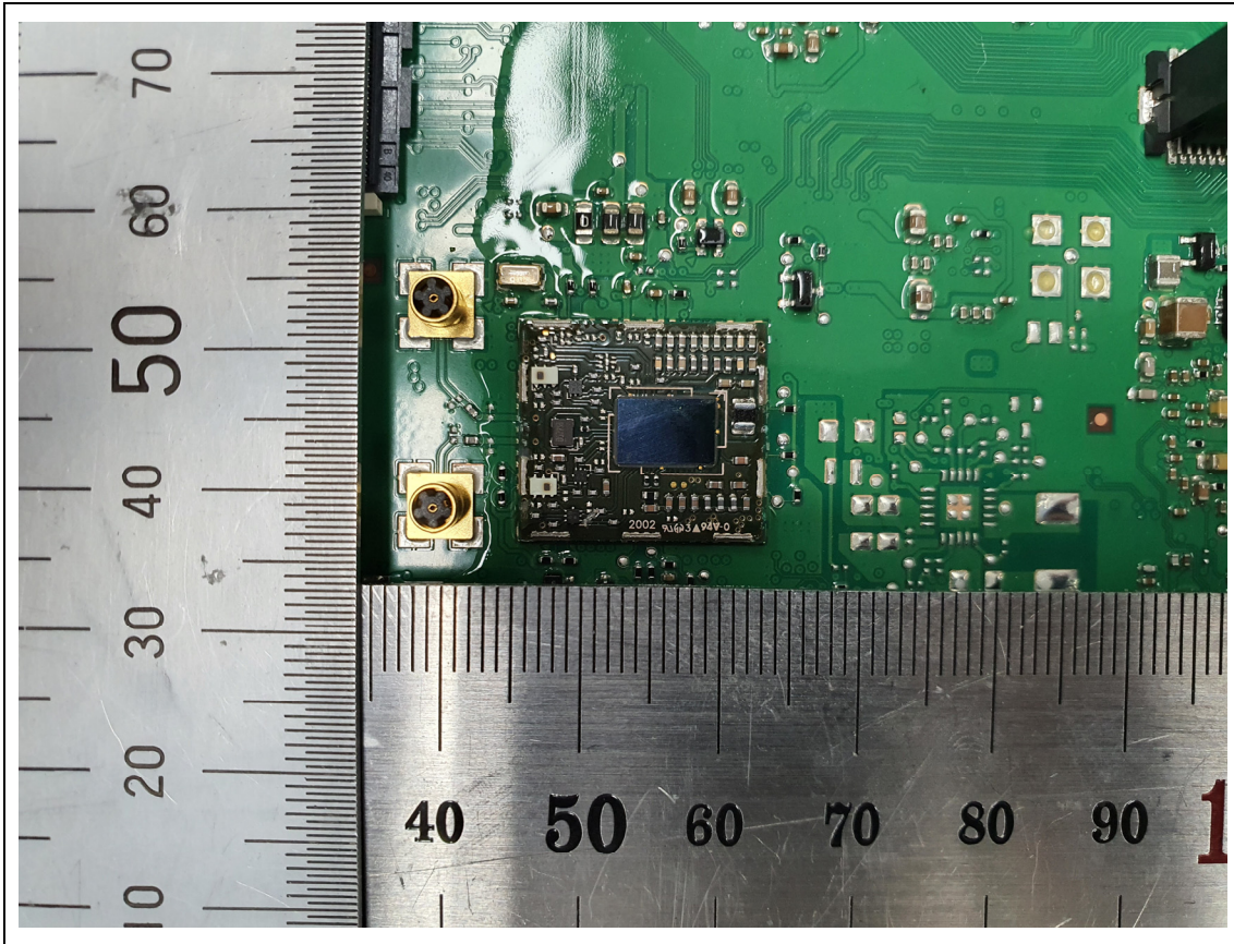
<BT,WiFi Module>
