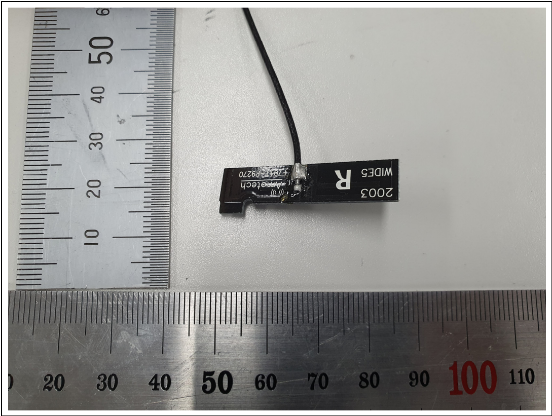
<Antenna 2>
