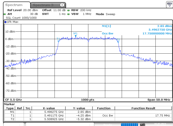
n20_5500MHz_Chain 0
