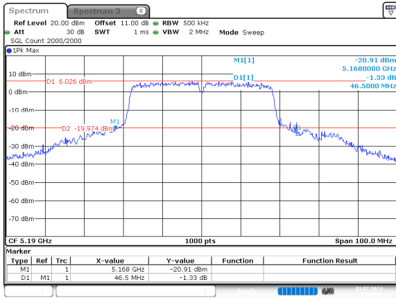
n40_5190MHz_Chain 0
