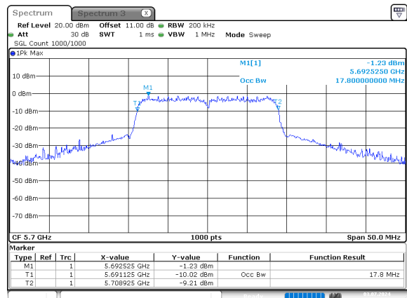
n20_5700MHz_Chain 0
