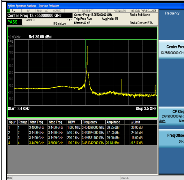
NTNV-n77(3450-3550)-PC2-30-50-L-CP-QPSK- Edge_1RB_Left-PASS
