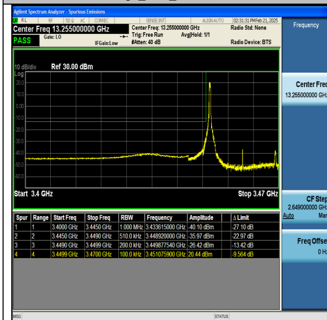
NTNV-n77(3450-3550)-PC2-30-20-L-CP-QPSK- Edge_1RB_Left-PASS
