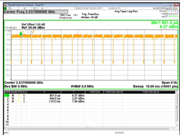
802.11n40
