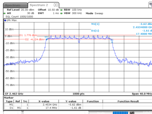
n20_2462MHz
