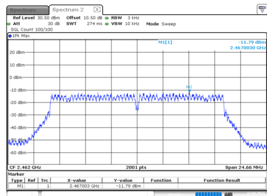
g_2462MHz
