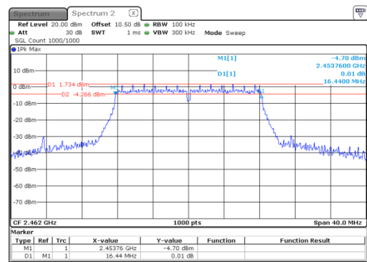
g_2462MHz
