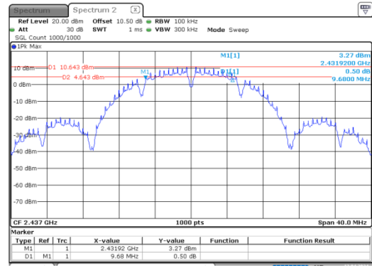
b_2437MHz
