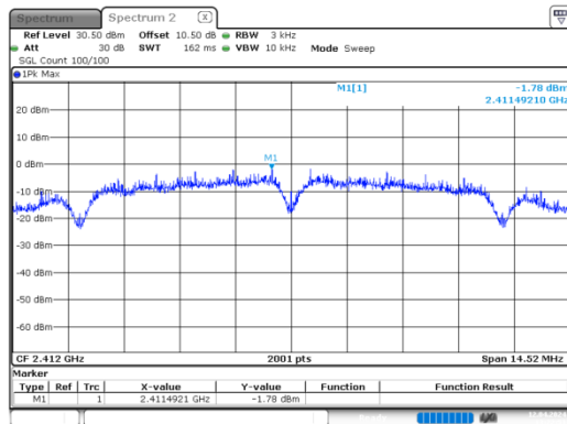
b_2412MHz
