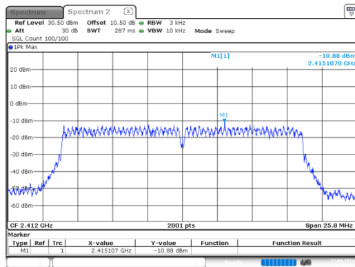
n20_2412MHz
