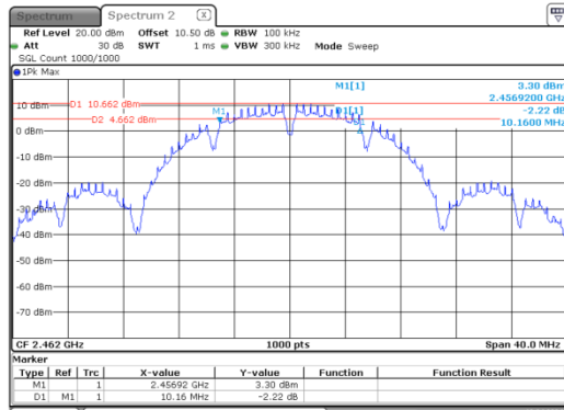
b_2462MHz
