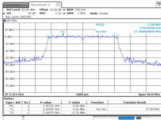
n20_2412MHz
