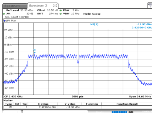
g_2437MHz
