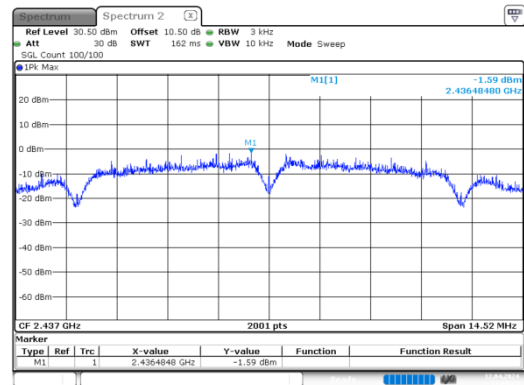
b_2437MHz
