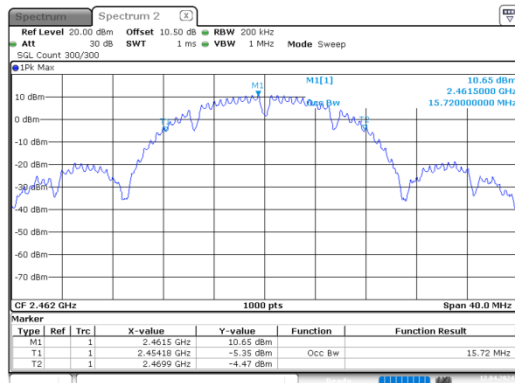
b_2462MHz
