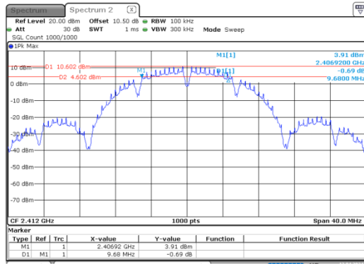
b_2412MHz
