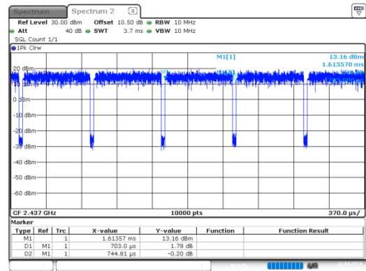
g_2437MHz
