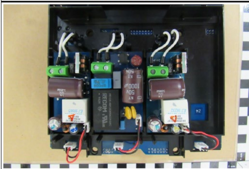
MULTICAL® 803 PCB
