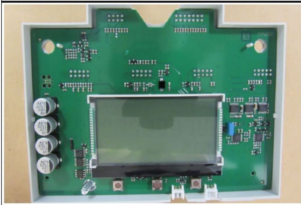
MULTICAL® 803 DISPLAY PCB
