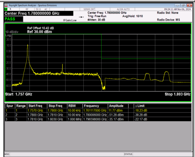
Band66-20MHz-QPSK-132572-100RB#0
