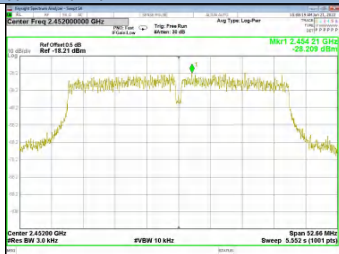
802.11n40 2452 MHz
