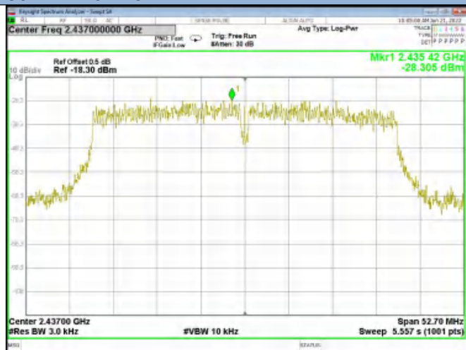
802.11n40 2437 MHz
