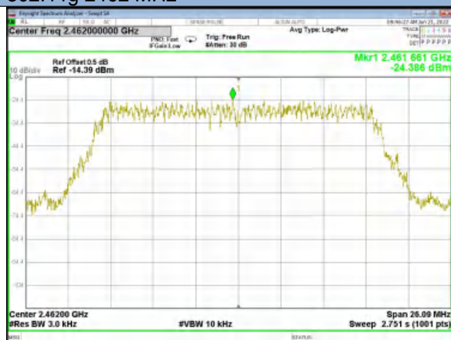
802.11g 2462 MHz
