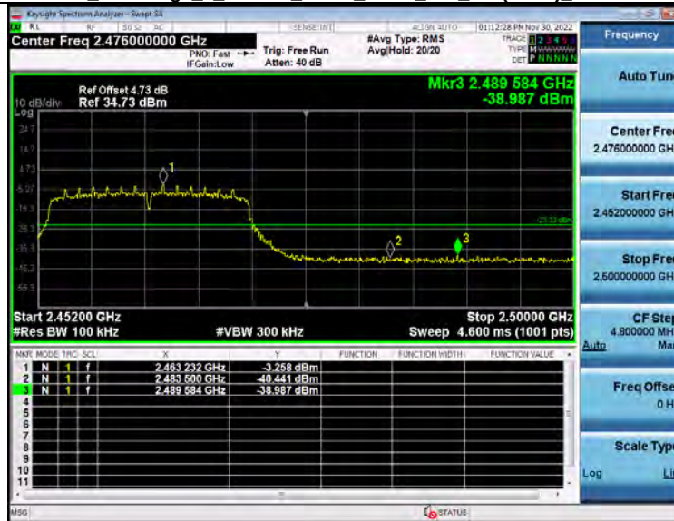
2_Bandedge 2 4GWiFi_NVNT ANT1 802 11n(HT20) 2462
