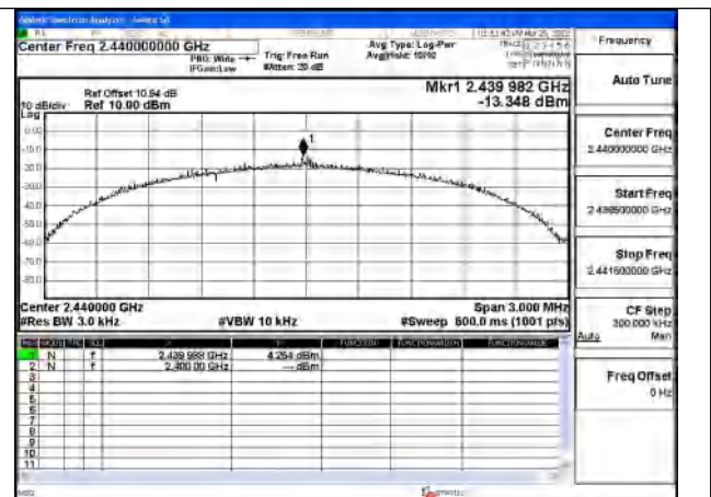
Test Mode:GFSK (LE 2Mbps) MHz
