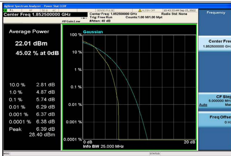
Band2-5MHz-16QAM-18625-1RB#0
