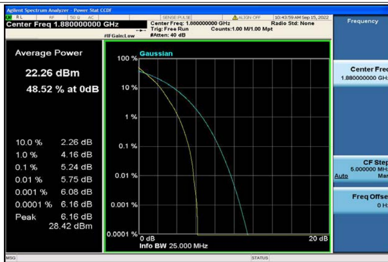
Band2-5MHz-QPSK-18900-25RB#0
