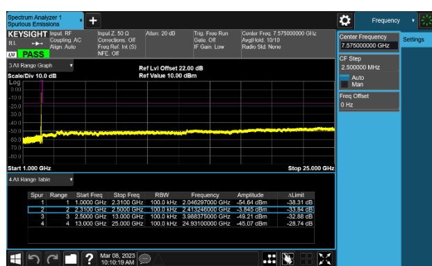
802.11 g CH01 (2412MHz)
