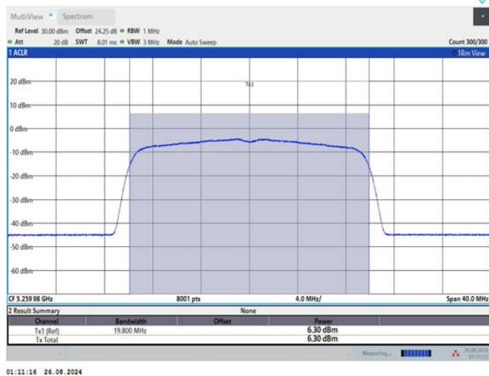
11AX20MIMO_Ant3_5260
