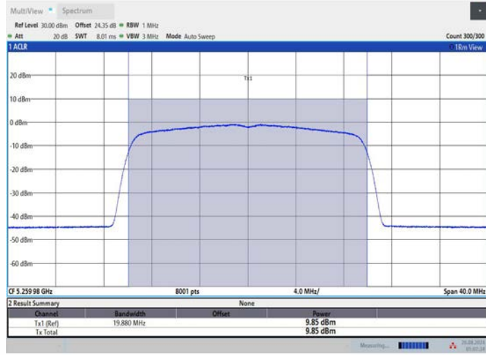
11AX20MIMO_Ant3_5260
