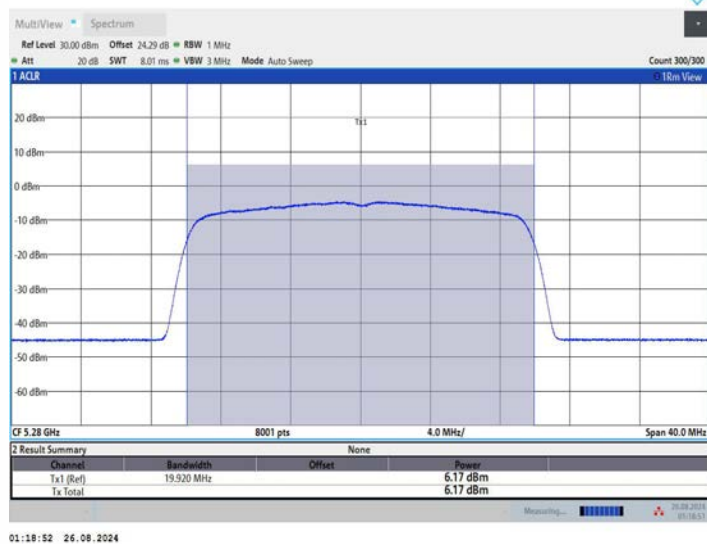
11AX20MIMO_Ant3_5280
