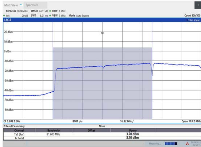
11AX160MIMO_Ant1_5250_UNII-1
