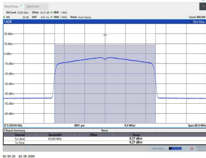
11AX40MIMO_Ant3_5550
