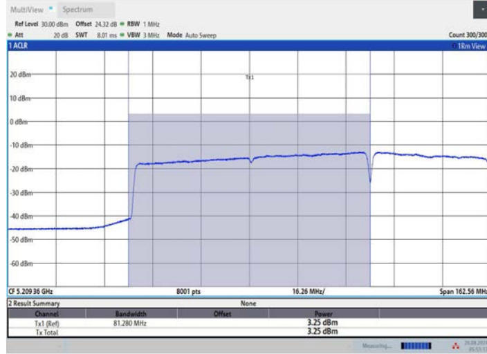
11AX160MIMO_Ant2_5250_UNII-1
