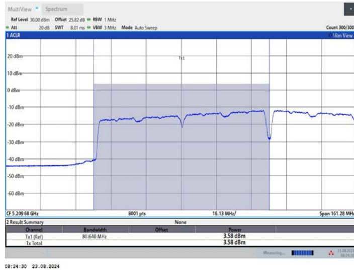
11AC160MIMO_Ant1_5250_UNII-1
