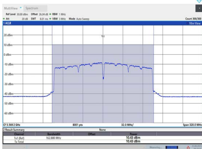
11AC160MIMO_Ant2_5570
