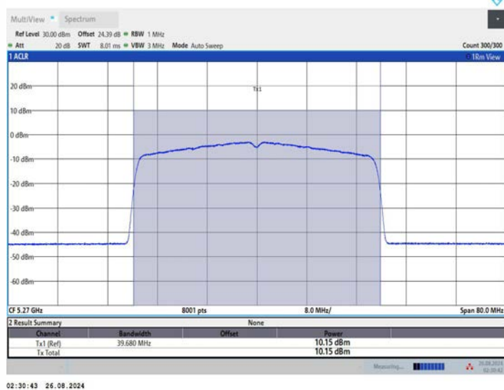
11AX40MIMO_Ant2_5270
