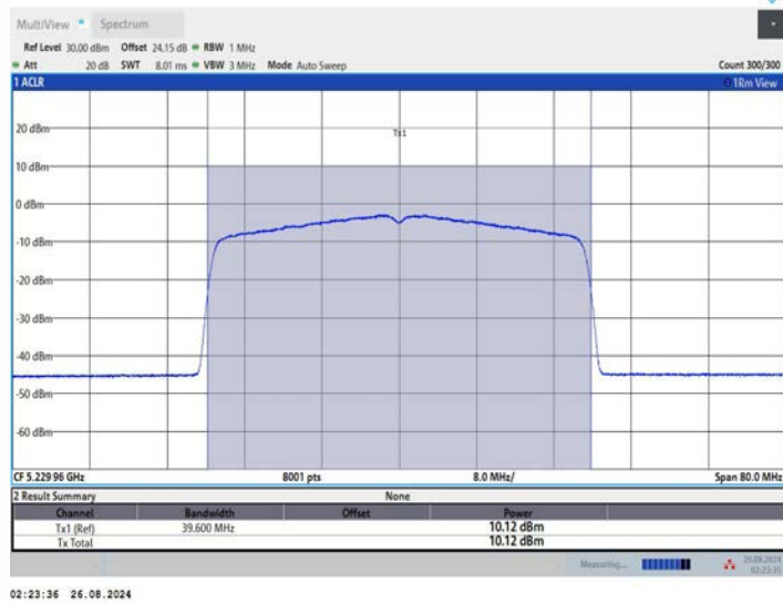
11AX40MIMO_Ant2_5230
