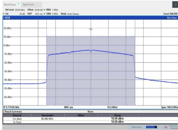
11AX80MIMO_Ant3_5775
