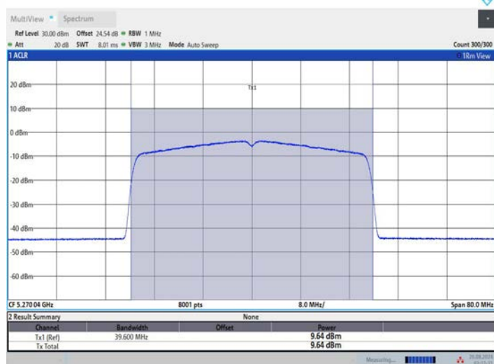
11AX40MIMO_Ant3_5270
