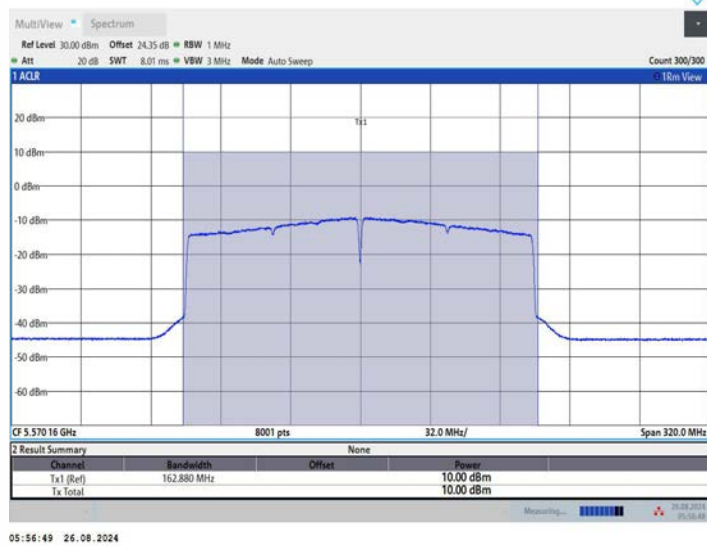
11AX160MIMO_Ant3_5570
