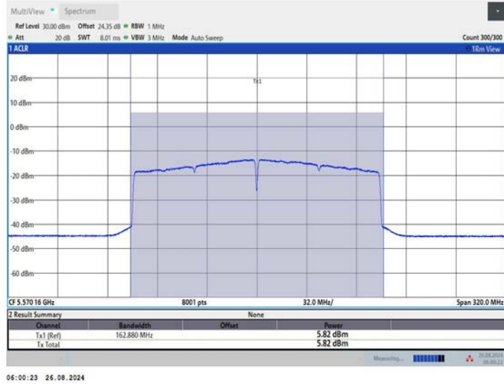
11AX160MIMO_Ant2_5570
