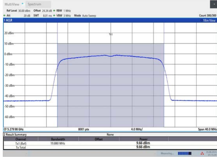
11AX20MIMO_Ant3_5280
