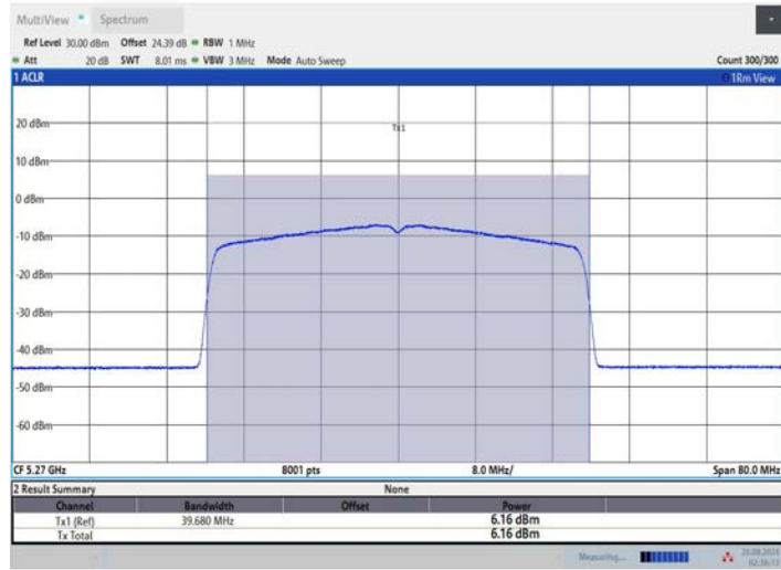
11AX40MIMO_Ant1_5270
