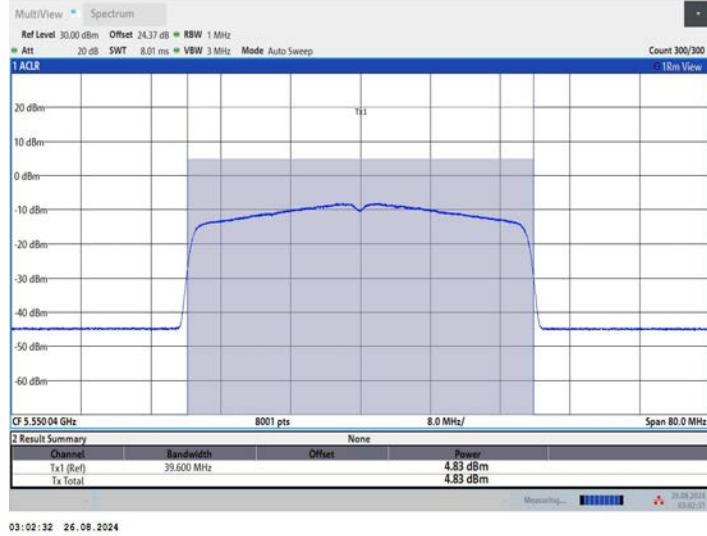
11AX40MIMO_Ant2_5550
