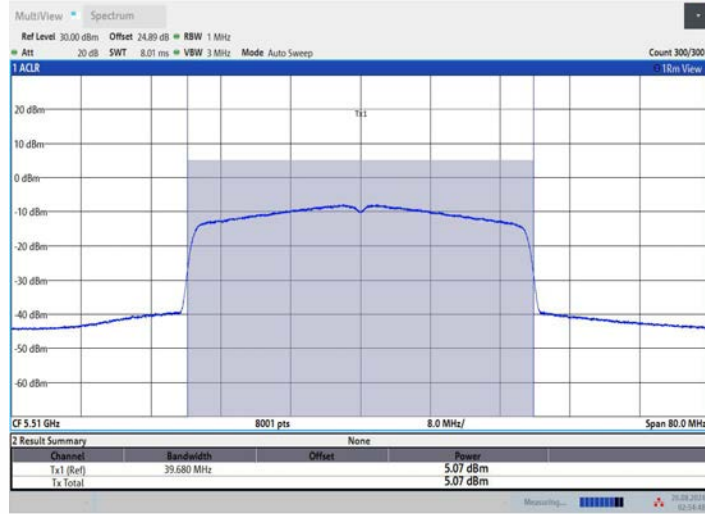
11AX40MIMO_Ant2_5510
