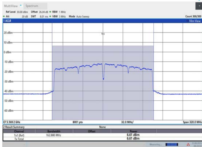
11AC160MIMO_Ant1_5570
