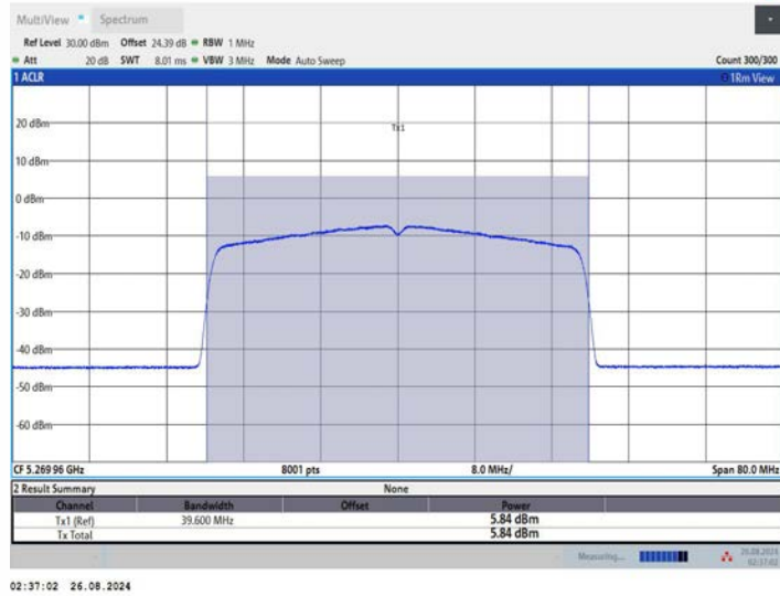
11AX40MIMO_Ant3_5270
