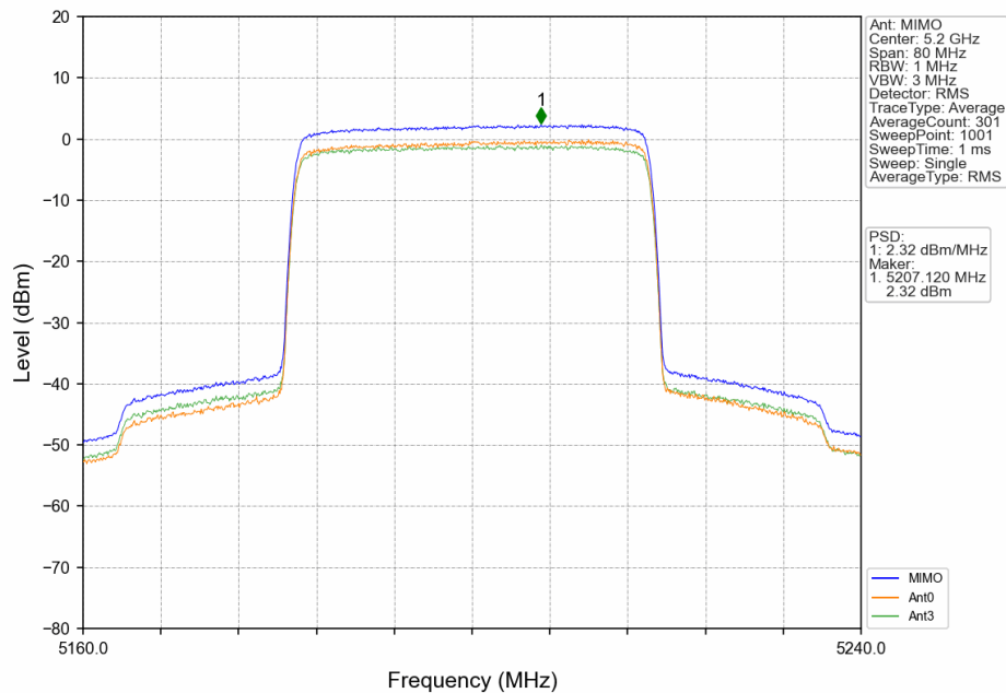
40_MCH_5200MHz_MIMO_NTNV
