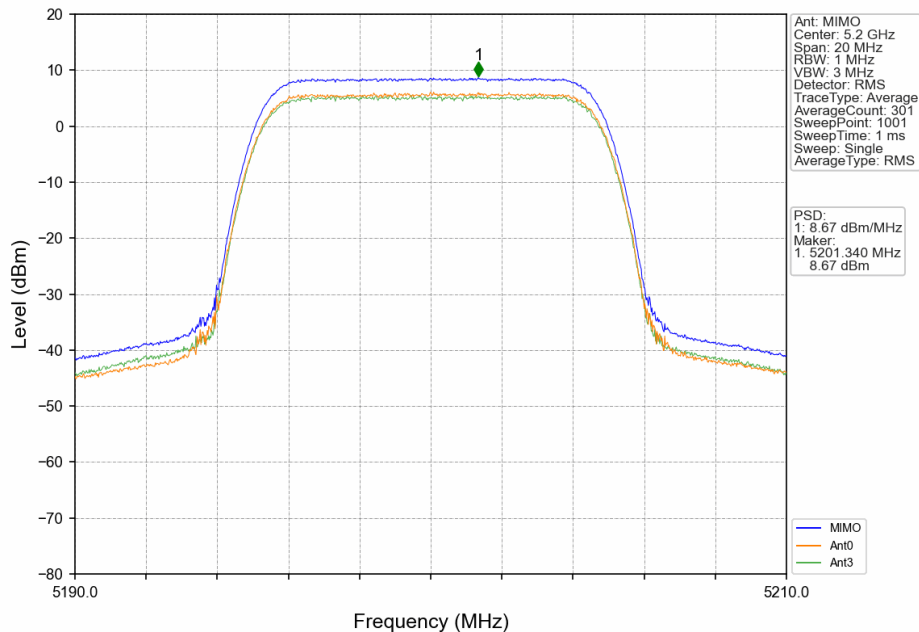
10_MCH_5200MHz_MIMO_NTNV
