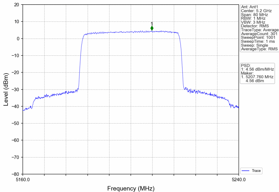
40_MCH_5200MHz_Ant1_NTNV
