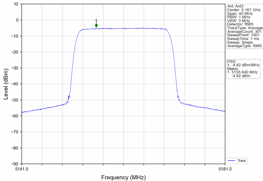
20_LCH_5161MHz_MIMO_NTNV
