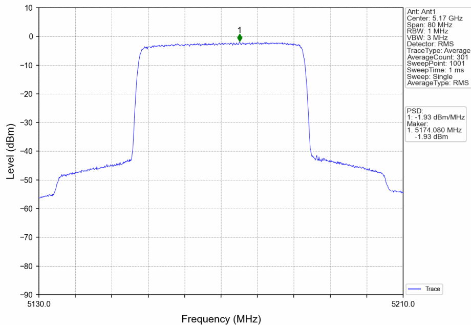
40_LCH_5170MHz_Ant1_NTNV
