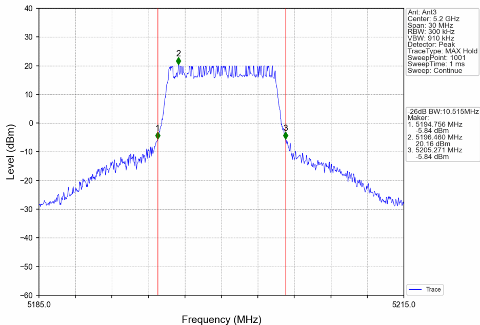
10_MCH_5200MHz_Ant3_NTNV
