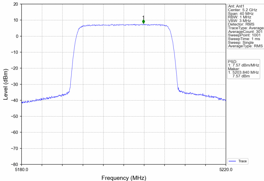
20_MCH_5200MHz_Ant1_NTNV
