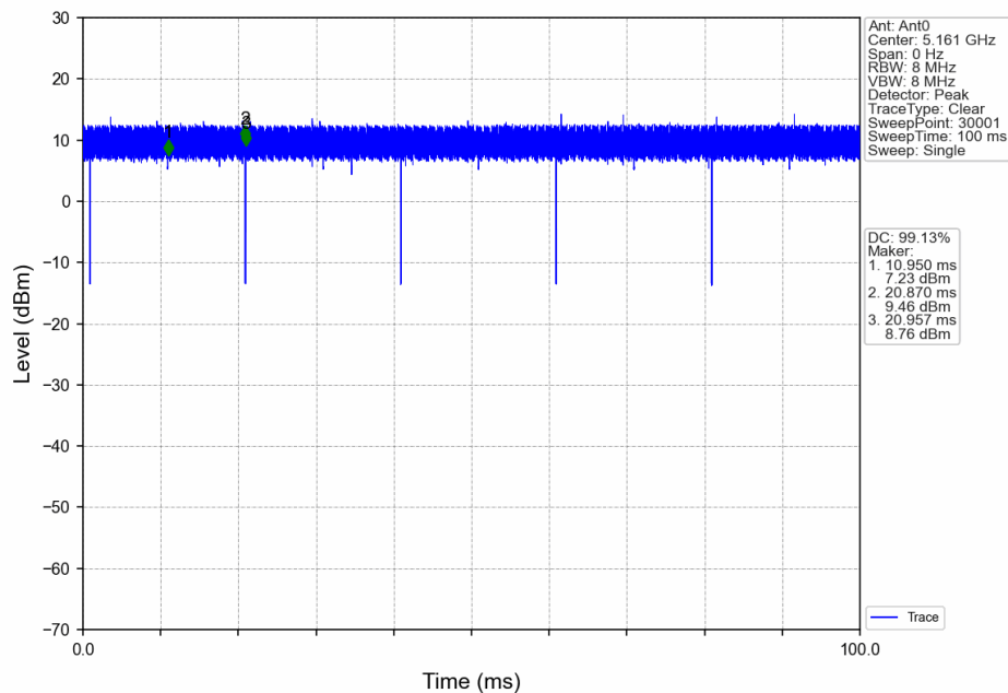
20_LCH_5161MHz_Ant0_NTNV
