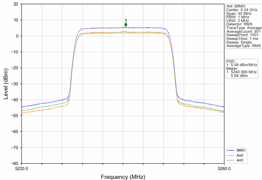
20_HCH_5240MHz_MIMO_NTNV
