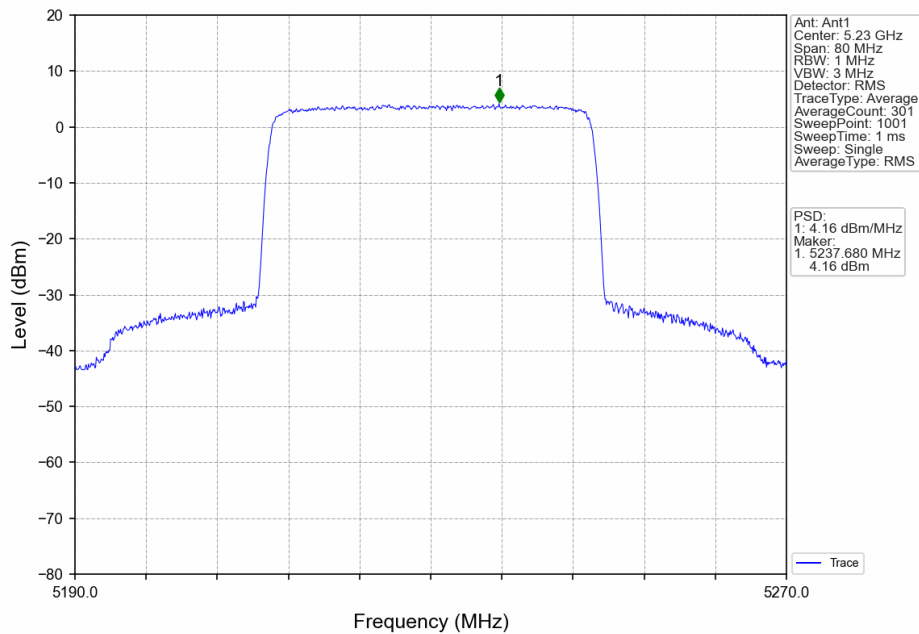
40_HCH_5230MHz_Ant1_NTNV
