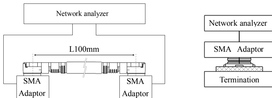
図 2. VSWR
