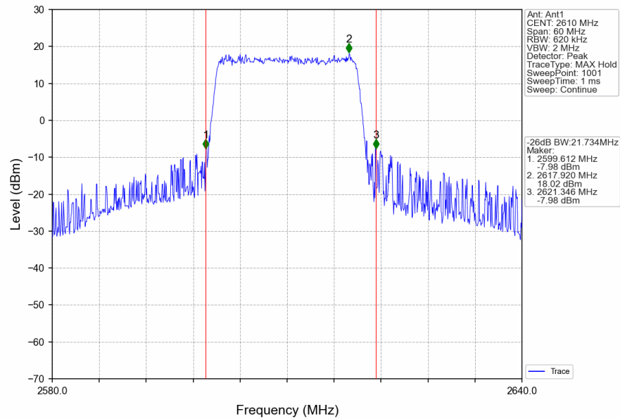
Band38_20MHz_16QAM_HCH_2610MHz_RB_100_0_NTNV
