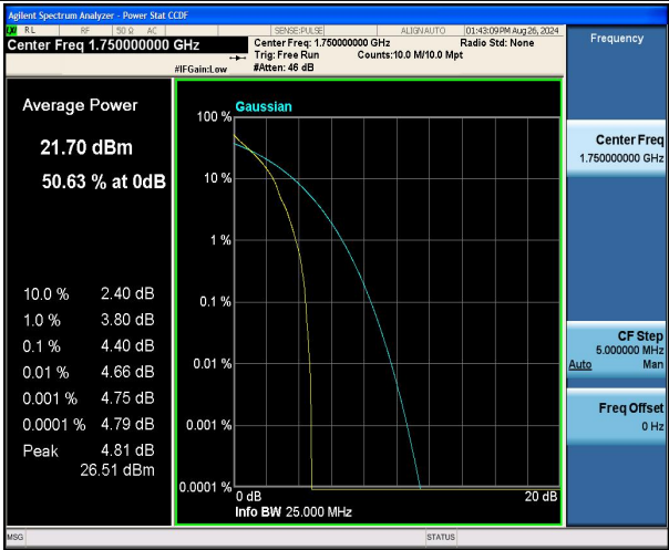
Band4-10MHz-QPSK-20350-1RB#0-PASS
