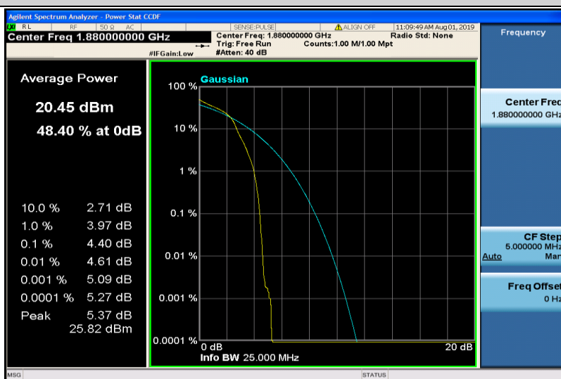
Band2-20MHz-16QAM-18900-1RB#0
