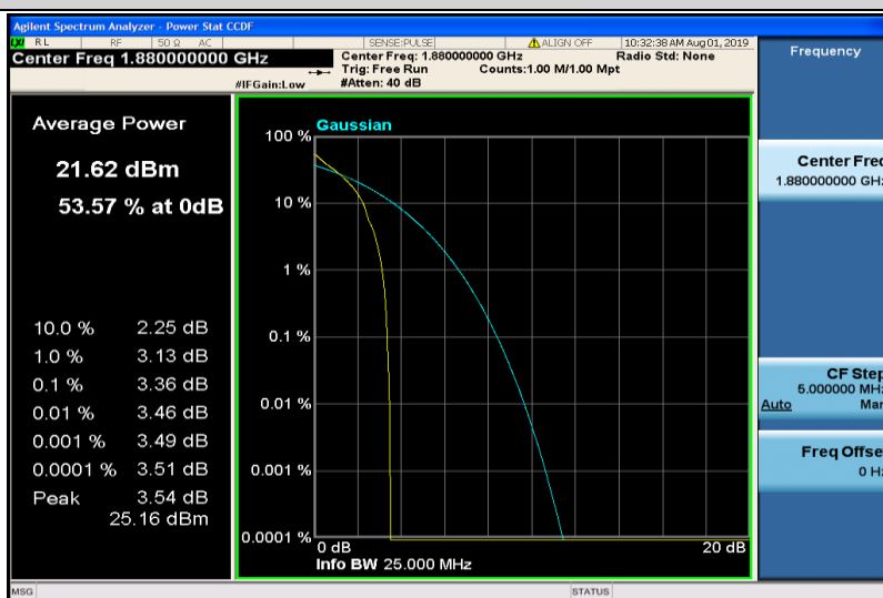
Band2-10MHz-QPSK-18900-1RB#0
