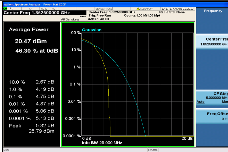
Band2-5MHz-16QAM-18625-1RB#0
