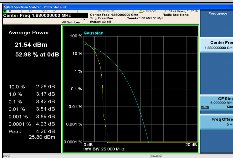
Band2-20MHz-QPSK-18900-1RB#0
