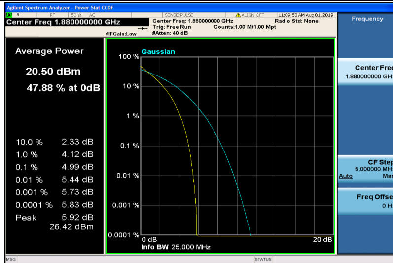
Band2-20MHz-QPSK-18900-100RB#0
