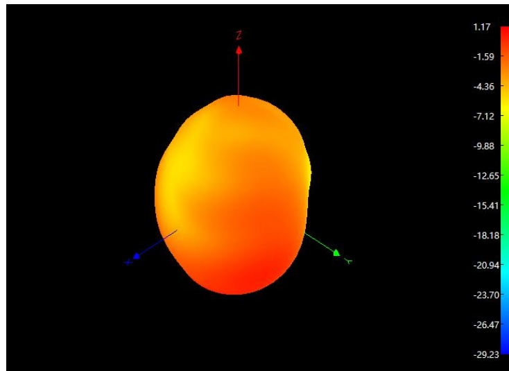
2500MHz 3D
