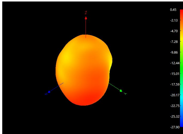
2450MHz 3D
