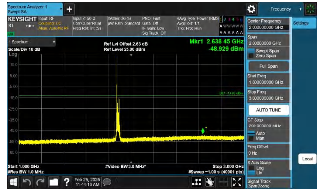
Band2-20MHz-QPSK-18900-1RB#0-1000~3000-PASS
