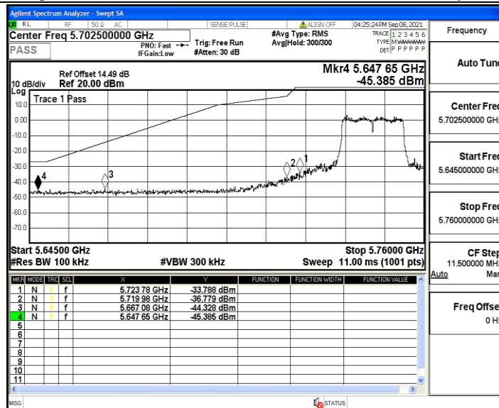
11AC20MIMO_Ant2_Low_5745
