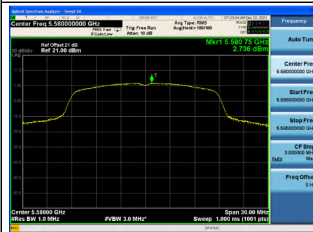
PSD_U-NII-2C_802.11n_5580
