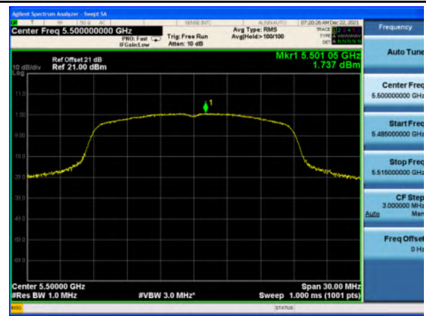
PSD_U-NII-2C_802.11n_5500
