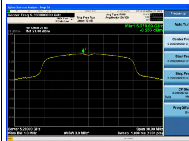
PSD_U-NII-2A_802.11n_5280
