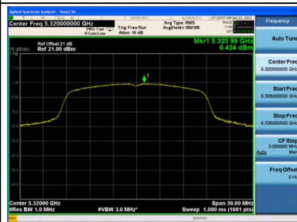
PSD_U-NII-2A_802.11n_5320
