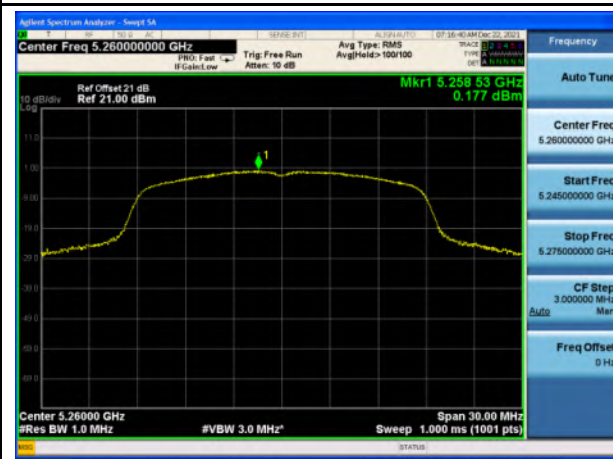
PSD_U-NII-2A_802.11n_5260
