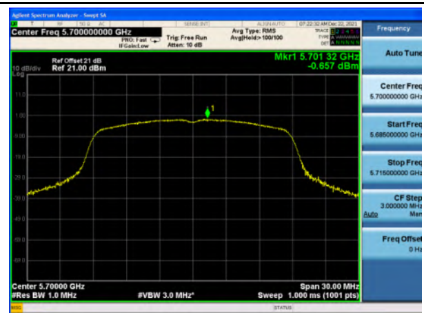
PSD_U-NII-2C_802.11n_5700
