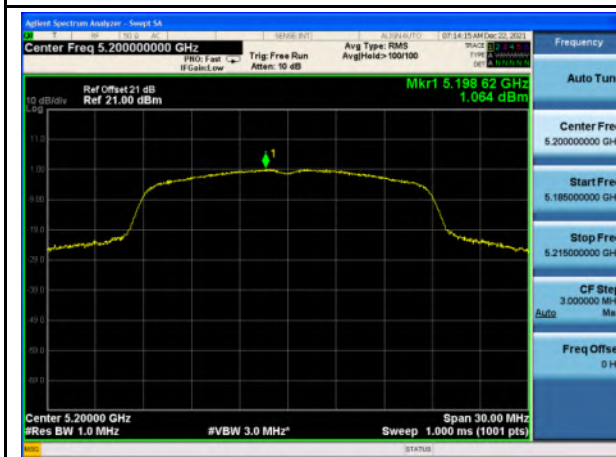
PSD_U-NII-1_802.11n_5200
