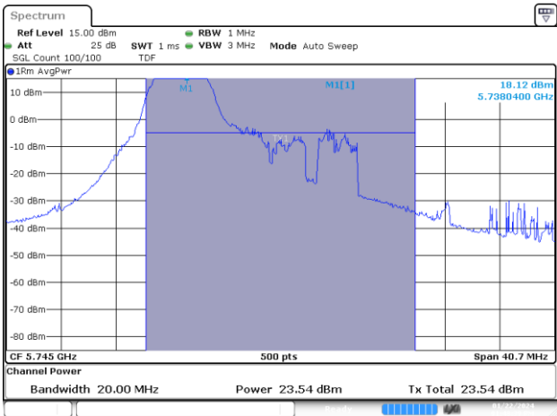
MIMO B-802.11ax/be20-CH149-MCS0 4m
