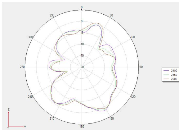
Phi 90 2D图
