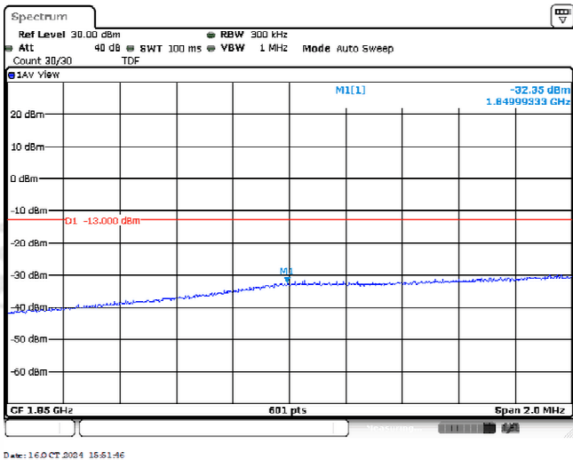
Band2-15MHz-16QAM-18675-1RB#24
