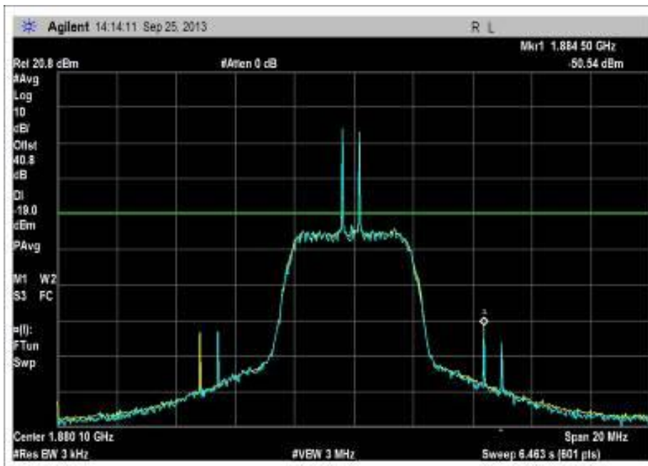
7.4 intermod_1850-1910MHz
