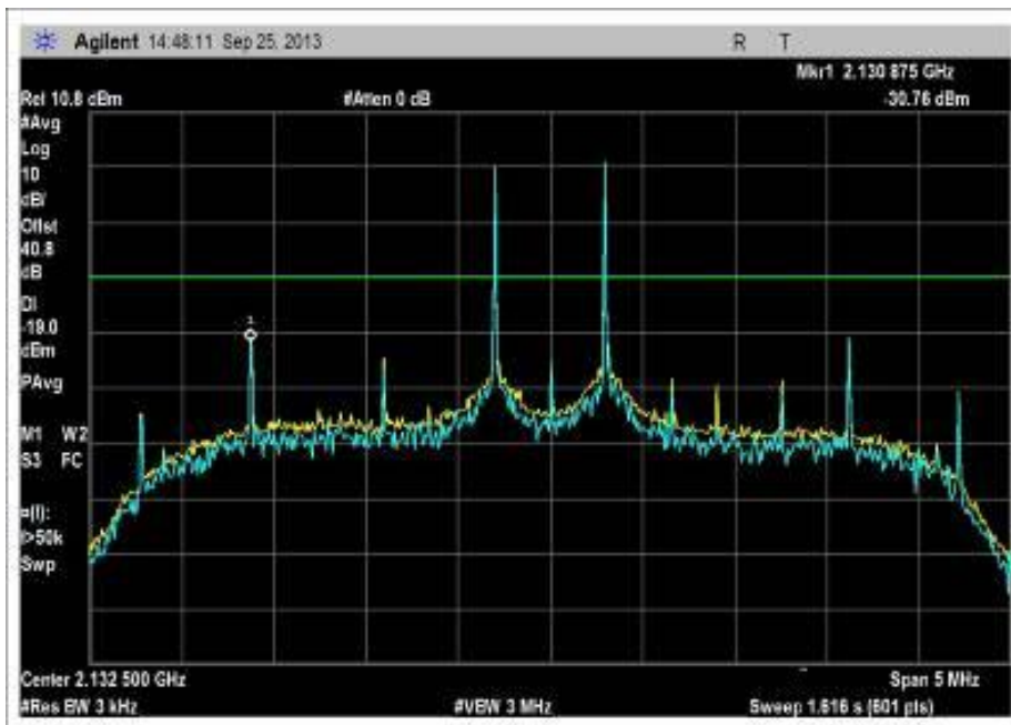
7.4 intermod_2110-2155MHz
