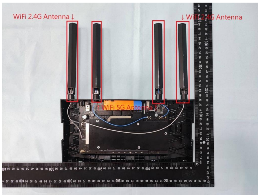
(2) EUT Photo
