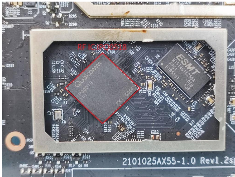
(10) EUT Photo
