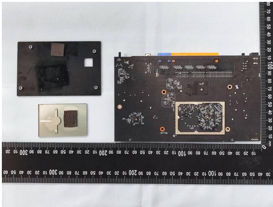
(14) EUT Photo
