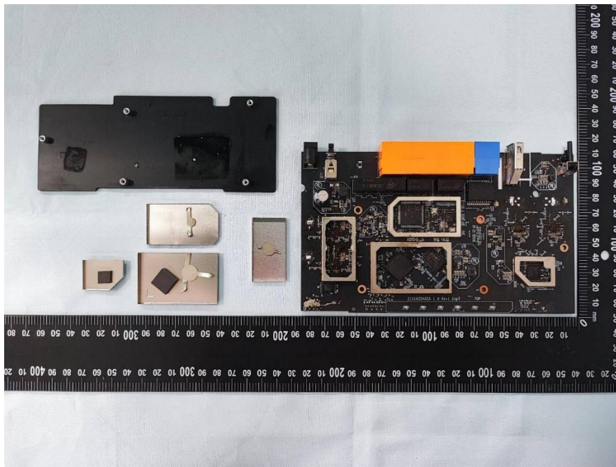
(6) EUT Photo
