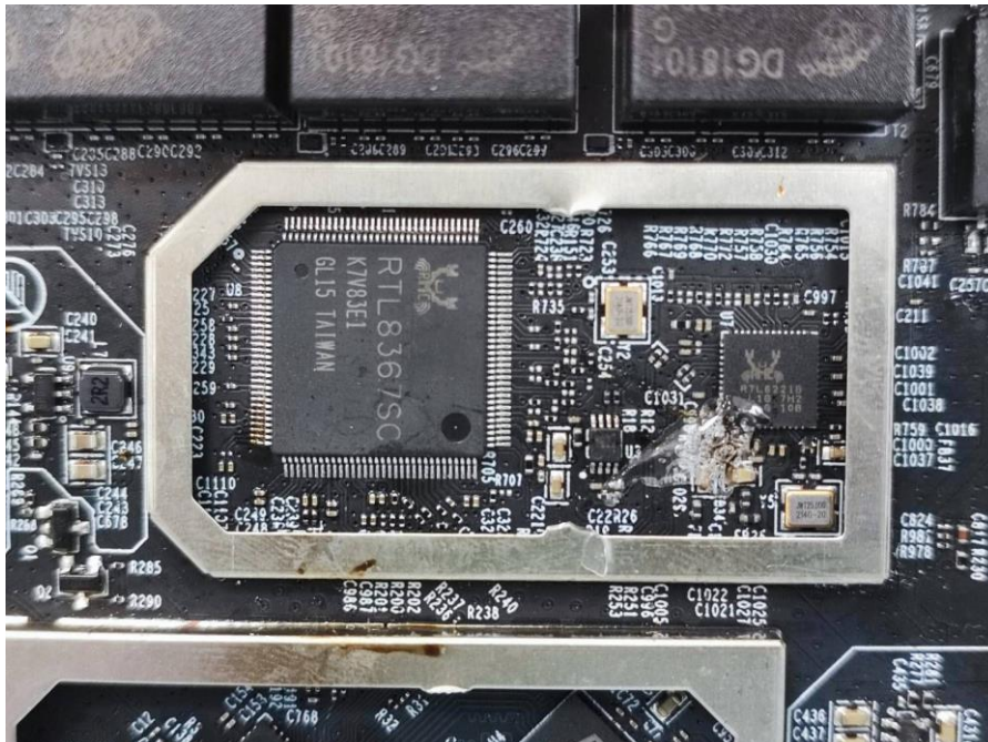
(8) EUT Photo
