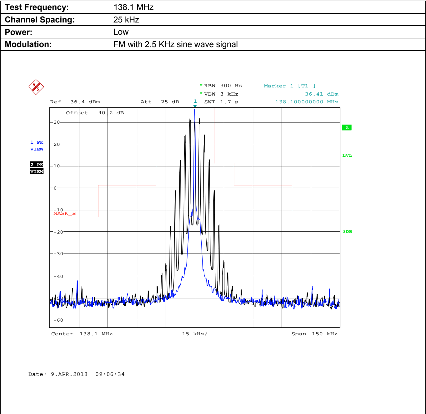
Plot 5.8.4.3.2. Emission Mask B, Low Power
