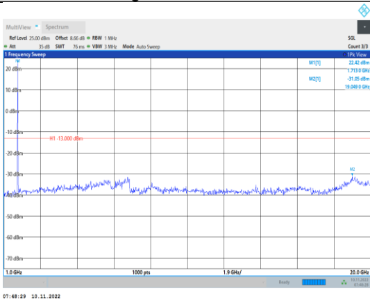
Band4-10MHz-QPSK-20000-1RB#0- Range2:1000~20000MHz
