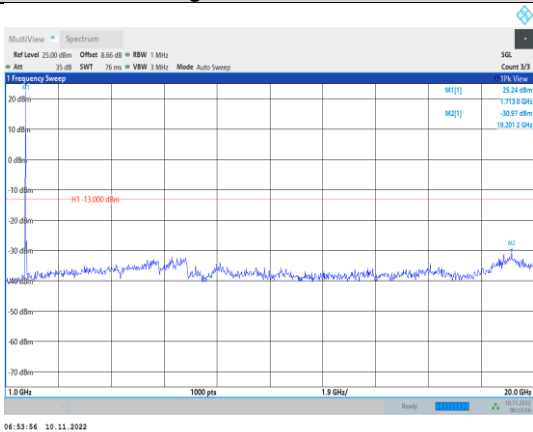
Band4-20MHz-QPSK-20050-1RB#0- Range2:1000~20000MHz
