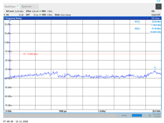
Band4-10MHz-QPSK-20175-1RB#0- Range2:1000~20000MHz
