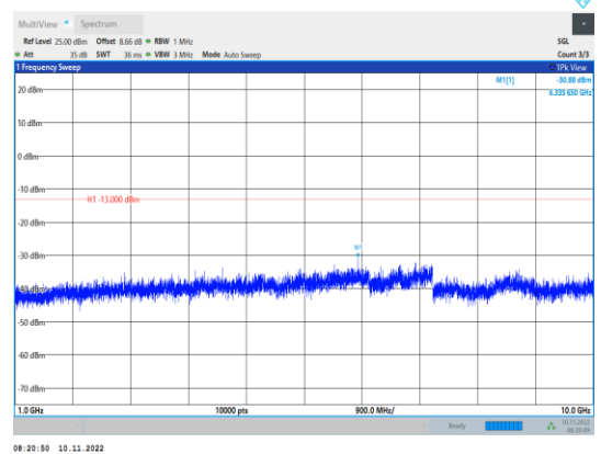
Band5-5MHz-QPSK-20525-1RB#0- Range2:1000~10000MHz
