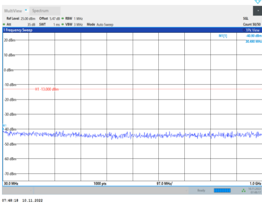
Band4-10MHz-QPSK-20000-1RB#0- Range1:30~1000MHz
