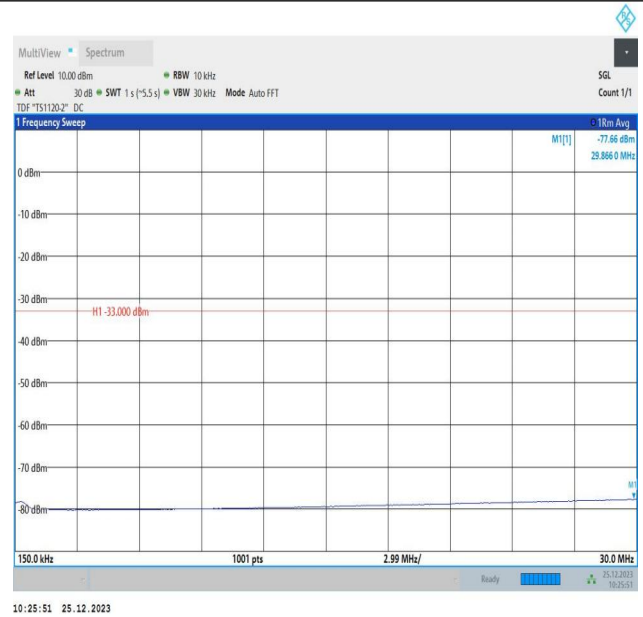
66-66-5MHz-10MHz-QPSK-QPSK-132375-132447-25RB#0-50RB#0-0.15~30MHz-PASS
