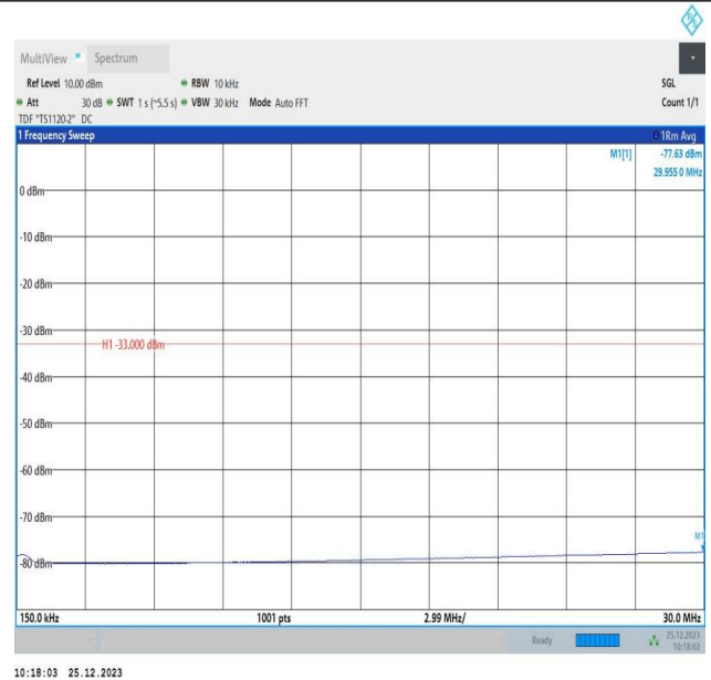
66-66-5MHz-10MHz-QPSK-QPSK-132000-132072-25RB#0-50RB#0-0.15~30MHz-PASS
