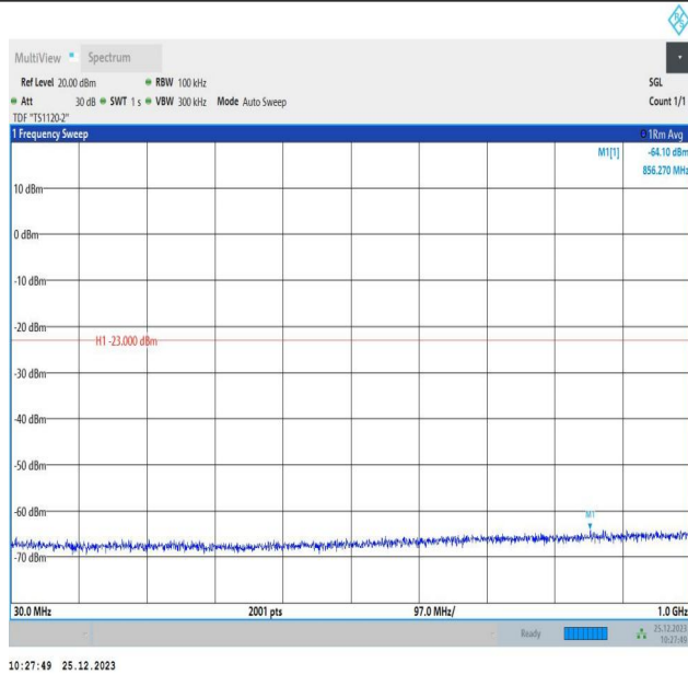
66-66-5MHz-10MHz-QPSK-QPSK-132550-132622-1RB#0-0 RB#0-30~1000MHz-PASS
