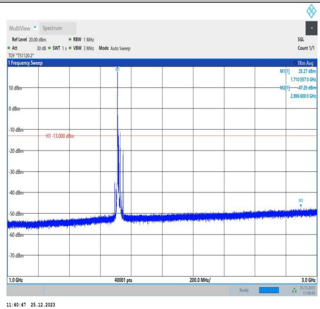
66-66-10MHz-5MHz-QPSK-QPSK-132022-132094-1RB#0-0R B#0-1000~3000MHz-PASS
