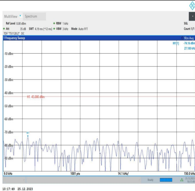
66-66-5MHz-10MHz-QPSK-QPSK-132000-132072-25RB#0-50RB#0-0.009~0.15MHz-PASS
