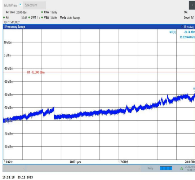
66-66-5MHz-10MHz-QPSK-QPSK-132375-132447-1RB#0-1 RB#49-3000~20000MHz-PASS
