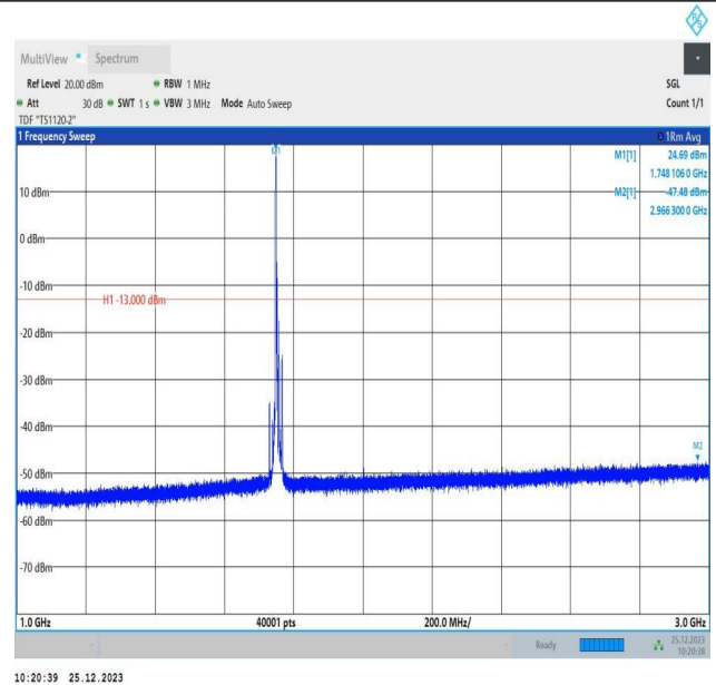
66-66-5MHz-10MHz-QPSK-QPSK-132375-132447-1RB#0-0R B#0-1000~3000MHz-PASS
