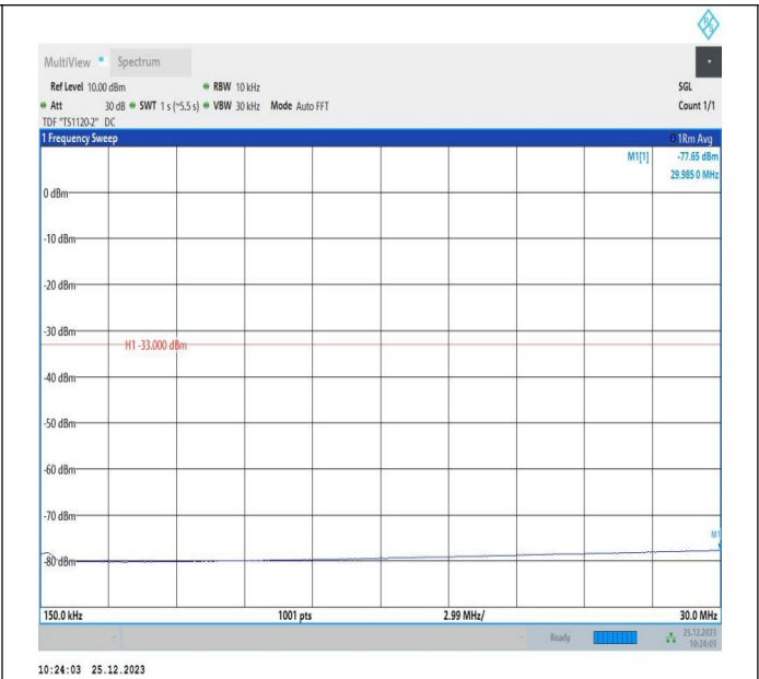
66-66-5MHz-10MHz-QPSK-QPSK-132375-132447-1RB#0-1R B#49-0.15~30MHz-PASS
