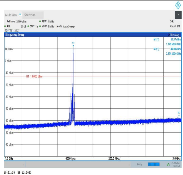
66-66-5MHz-10MHz-QPSK-QPSK-132550-132622-1RB#0-1R B#49-1000~3000MHz-PASS
