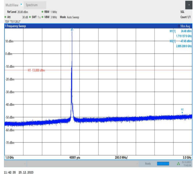
66-66-10MHz-5MHz-QPSK-QPSK-132022-132094-1RB#49-0 RB#0-1000~3000MHz-PASS
