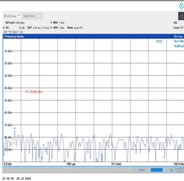
66-66-5MHz-10MHz-QPSK-QPSK-132550-132622-25RB#0-50RB#0-0.009~0.15MHz-PASS
