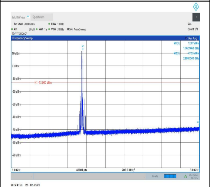
66-66-5MHz-10MHz-QPSK-QPSK-132375-132447-1RB#0-1R B#49-1000~3000MHz-PASS
