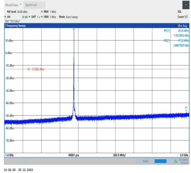
66-66-5MHz-10MHz-QPSK-QPSK-132375-132447-1RB#24-0 RB#0-1000~3000MHz-PASS
