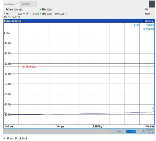
66-66-5MHz-10MHz-QPSK-QPSK-132550-132622-1RB#0-0R B#0-0.15~30MHz-PASS
