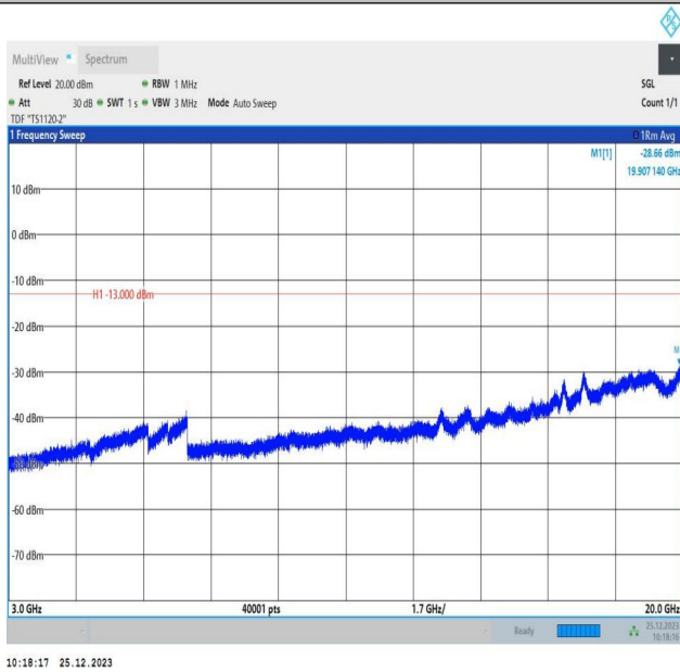
66-66-5MHz-10MHz-QPSK-QPSK-132000-132072-25RB#0-50RB#0-3000~20000MHz-PASS
