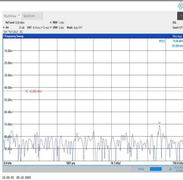
66-66-5MHz-10MHz-QPSK-QPSK-132375-132447-1RB#24-0RB#0-0.009~0.15MHz-PASS
