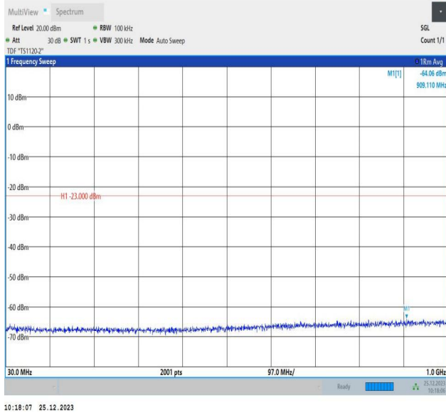
66-66-5MHz-10MHz-QPSK-QPSK-132000-132072-25RB#0-50RB#0-30~1000MHz-PASS
