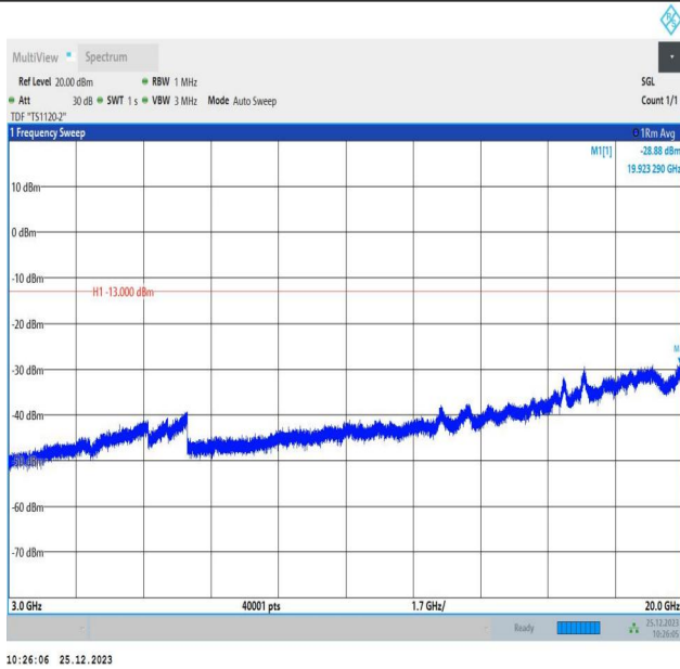
66-66-5MHz-10MHz-QPSK-QPSK-132375-132447-25RB#0-50RB#0-3000~20000MHz-PASS
