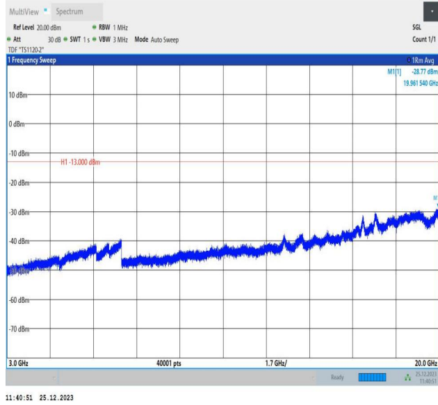
66-66-10MHz-5MHz-QPSK-QPSK-132022-132094-1RB#0-0RB#0-3000~20000MHz-PASS
