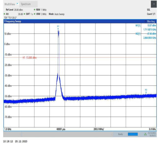
66-66-5MHz-10MHz-QPSK-QPSK-132000-132072-25RB#0-50RB#0-1000~3000MHz-PASS
