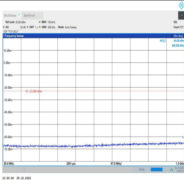
66-66-5MHz-10MHz-QPSK-QPSK-132375-132447-1RB#0-0 RB#0-30~1000MHz-PASS
