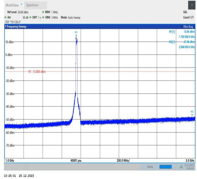
66-66-5MHz-10MHz-QPSK-QPSK-132375-132447-25RB#0-50RB#0-1000~3000MHz-PASS
