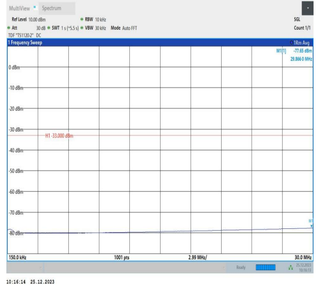
66-66-5MHz-10MHz-QPSK-QPSK-132000-132072-1RB#0-1R B#49-0.15~30MHz-PASS
