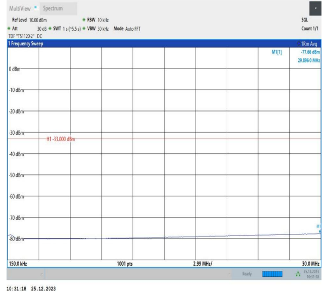
66-66-5MHz-10MHz-QPSK-QPSK-132550-132622-1RB#0-1R B#49-0.15~30MHz-PASS
