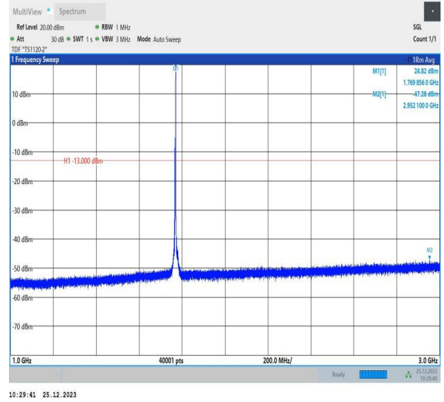
66-66-5MHz-10MHz-QPSK-QPSK-132550-132622-1RB#24-0 RB#0-1000~3000MHz-PASS
