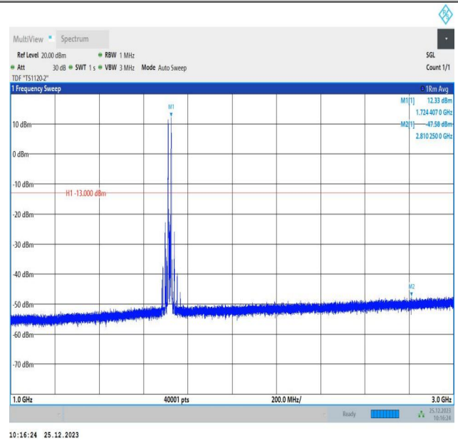
66-66-5MHz-10MHz-QPSK-QPSK-132000-132072-1RB#0-1R B#49-1000~3000MHz-PASS
