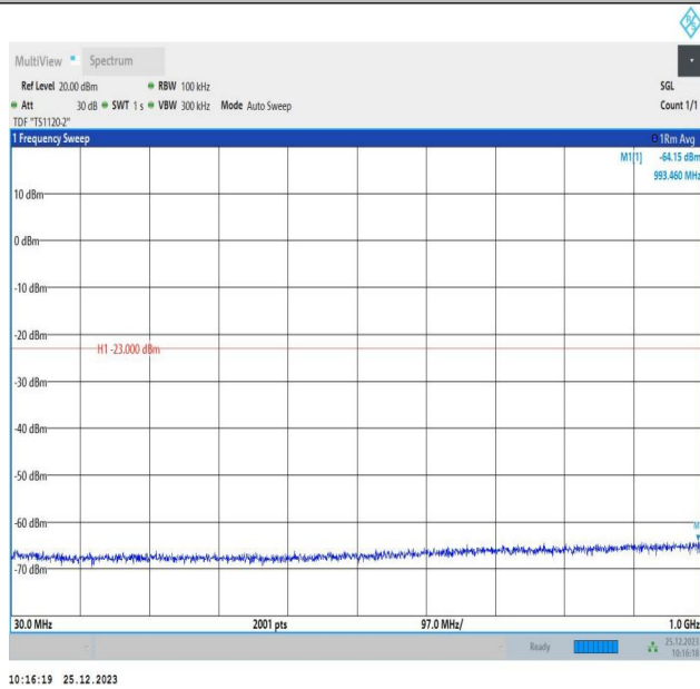
66-66-5MHz-10MHz-QPSK-QPSK-132000-132072-1RB#0-1 RB#49-30~1000MHz-PASS
