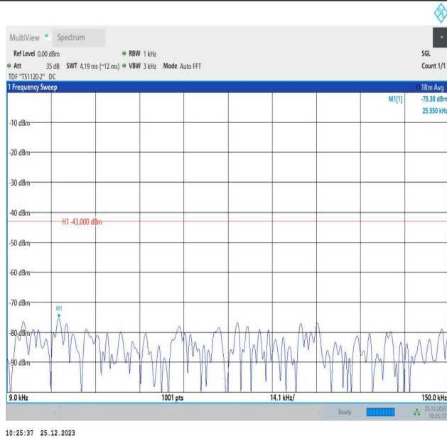
66-66-5MHz-10MHz-QPSK-QPSK-132375-132447-25RB#0-50RB#0-0.009~0.15MHz-PASS
