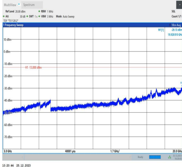
66-66-5MHz-10MHz-QPSK-QPSK-132375-132447-1RB#0-0 RB#0-3000~20000MHz-PASS
