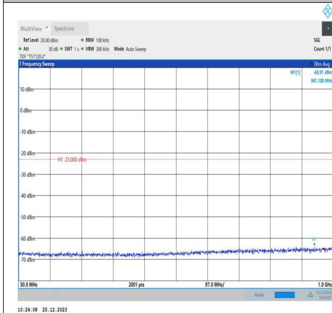
66-66-5MHz-10MHz-QPSK-QPSK-132375-132447-1RB#0-1 RB#49-30~1000MHz-PASS
