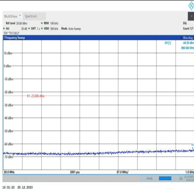
66-66-5MHz-10MHz-QPSK-QPSK-132550-132622-1RB#0-1 RB#49-30~1000MHz-PASS
