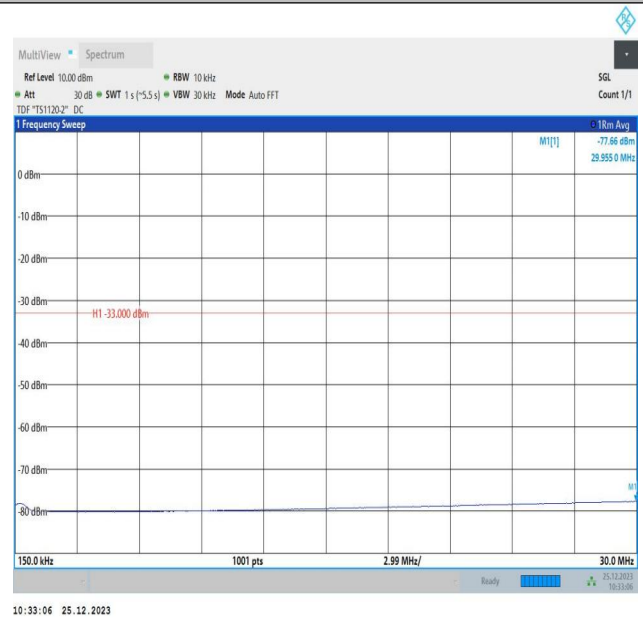
66-66-5MHz-10MHz-QPSK-QPSK-132550-132622-25RB#0-50RB#0-0.15~30MHz-PASS
