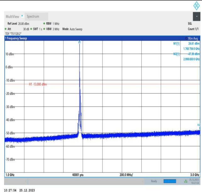
66-66-5MHz-10MHz-QPSK-QPSK-132550-132622-1RB#0-0R B#0-1000~3000MHz-PASS
