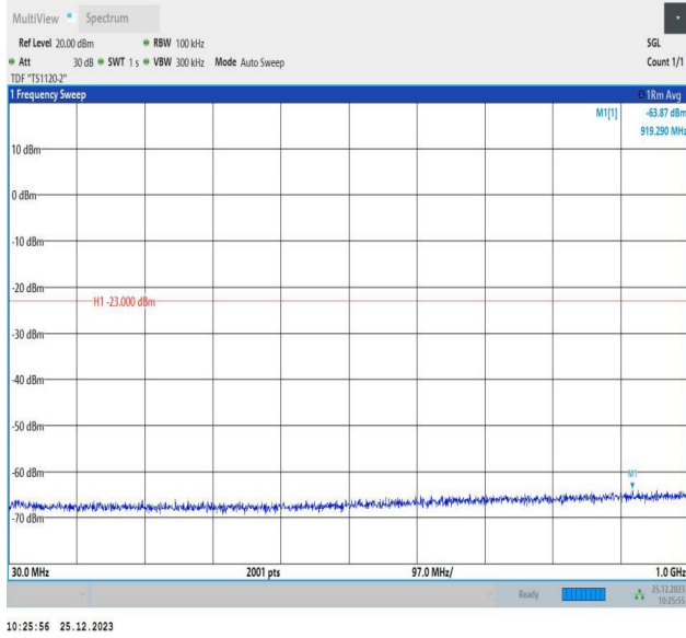
66-66-5MHz-10MHz-QPSK-QPSK-132375-132447-25RB#0-50RB#0-30~1000MHz-PASS
