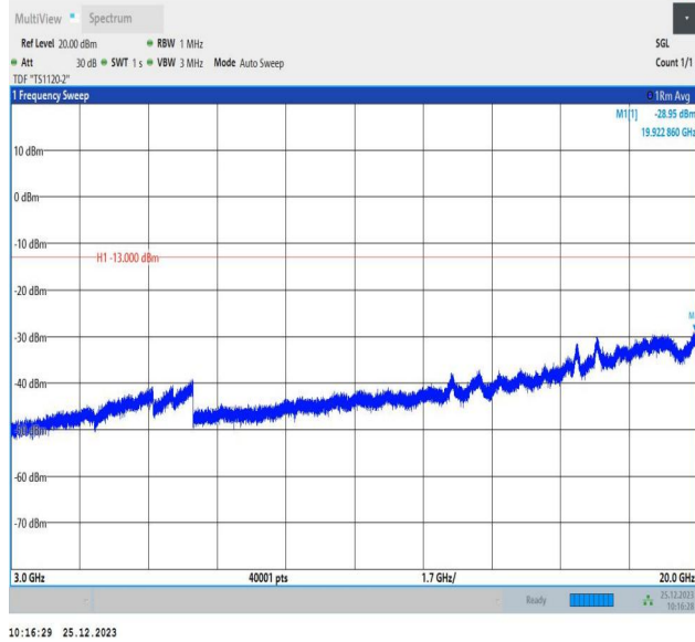
66-66-5MHz-10MHz-QPSK-QPSK-132000-132072-1RB#0-1 RB#49-3000~20000MHz-PASS
