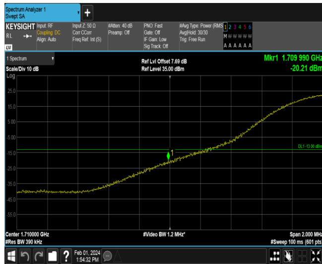
Band66-20MHz-16QAM-132072-1RB#99
