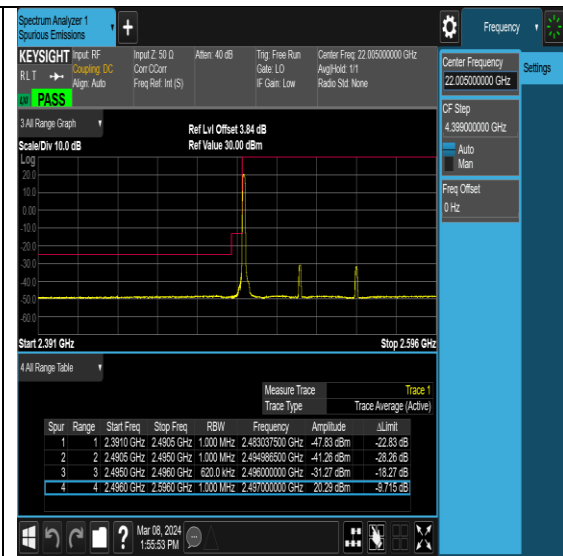
NTNV-N41-PC2-30-60-L-DFT-QPSK-Edge_1RB_Left-Ant0-PASS
