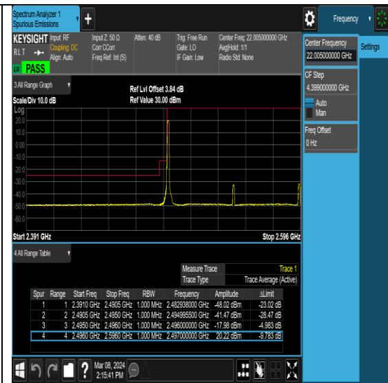
NTNV-N41-PC2-30-100-L-DFT-QPSK-Edge_1RB_Left-Ant0-PASS
