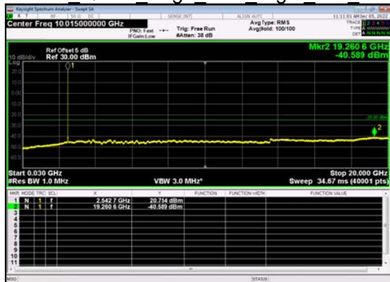
N7(15M)_DFT-s- OFDM QPSK Edge 1RB Right Mid CH
