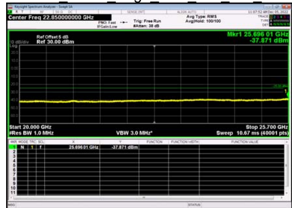
N7(15M)_DFT-s- OFDM BPSK Edge 1RB Left Mid CH
