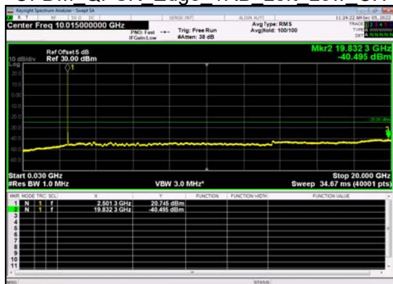
N7(20M)_DFT-s- OFDM QPSK Edge 1RB Left Low CH
