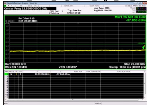
N7(15M)_DFT-s- OFDM BPSK Edge 1RB Right Mid CH
