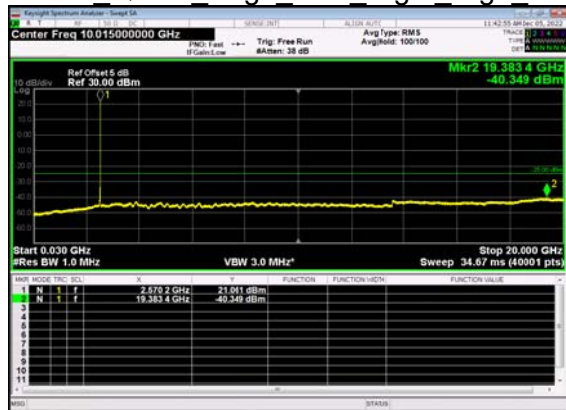
N7(20M)_DFT-s- OFDM QPSK Edge 1RB Right High CH
