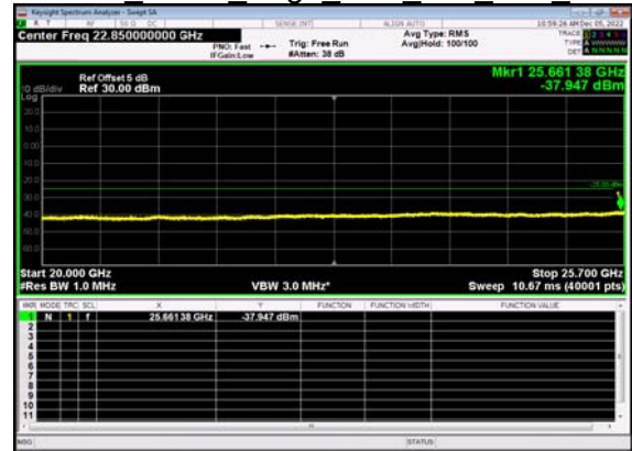
N7(15M)_DFT-s- OFDM BPSK Edge 1RB Left Low CH
