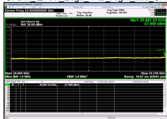
N7(20M)_DFT-s- OFDM QPSK Edge 1RB Right Mid CH
