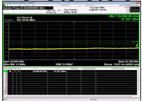
N7(20M)_DFT-s- OFDM QPSK Edge 1RB Right Low CH
