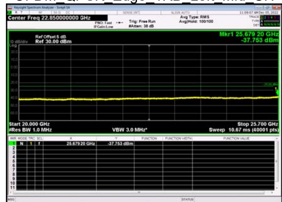
N7(15M)_DFT-s- OFDM QPSK Edge 1RB Left Mid CH
