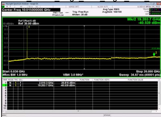
N7(15M)_DFT-s- OFDM QPSK Edge 1RB Right Low CH
