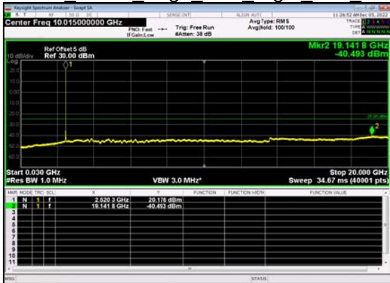
N7(20M)_DFT-s- OFDM QPSK Edge 1RB Right Low CH
