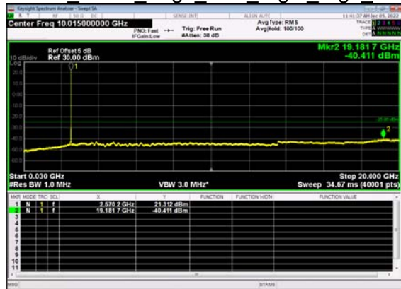
N7(20M)_DFT-s- OFDM BPSK Edge 1RB Right High CH
