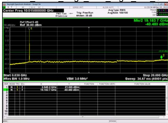
N7(20M)_DFT-s- OFDM BPSK Edge 1RB Right Mid CH
