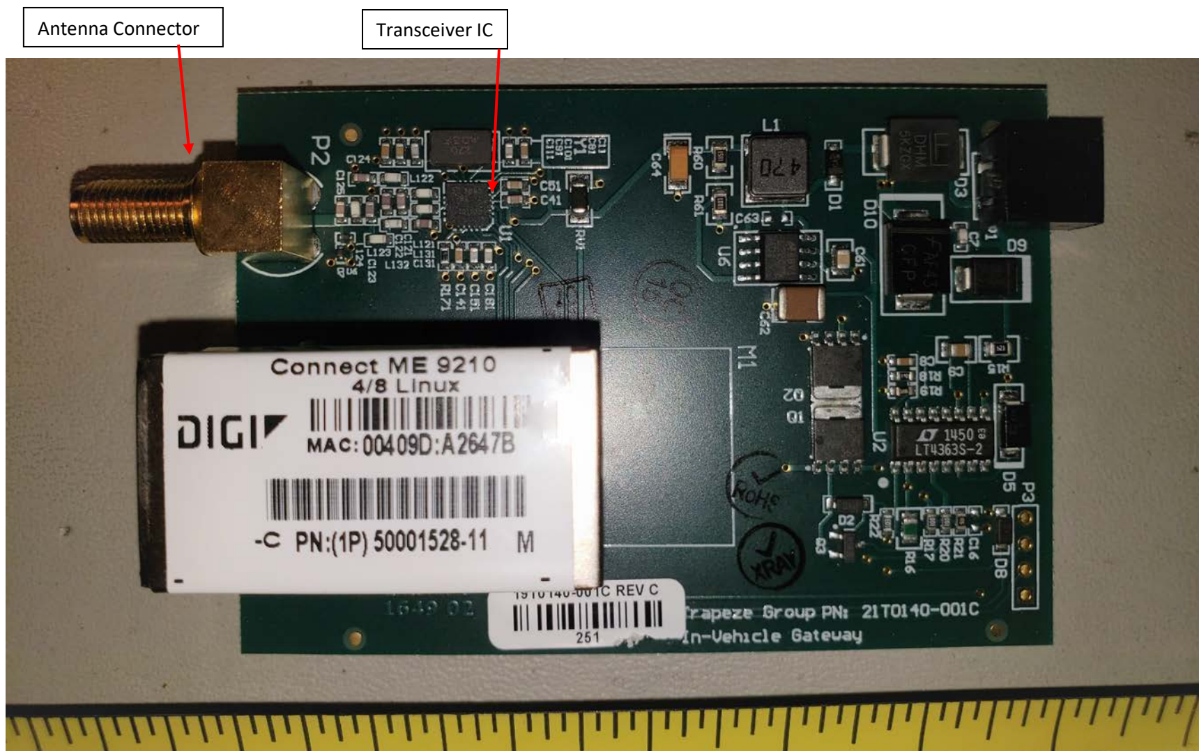
PCBA Top Side
