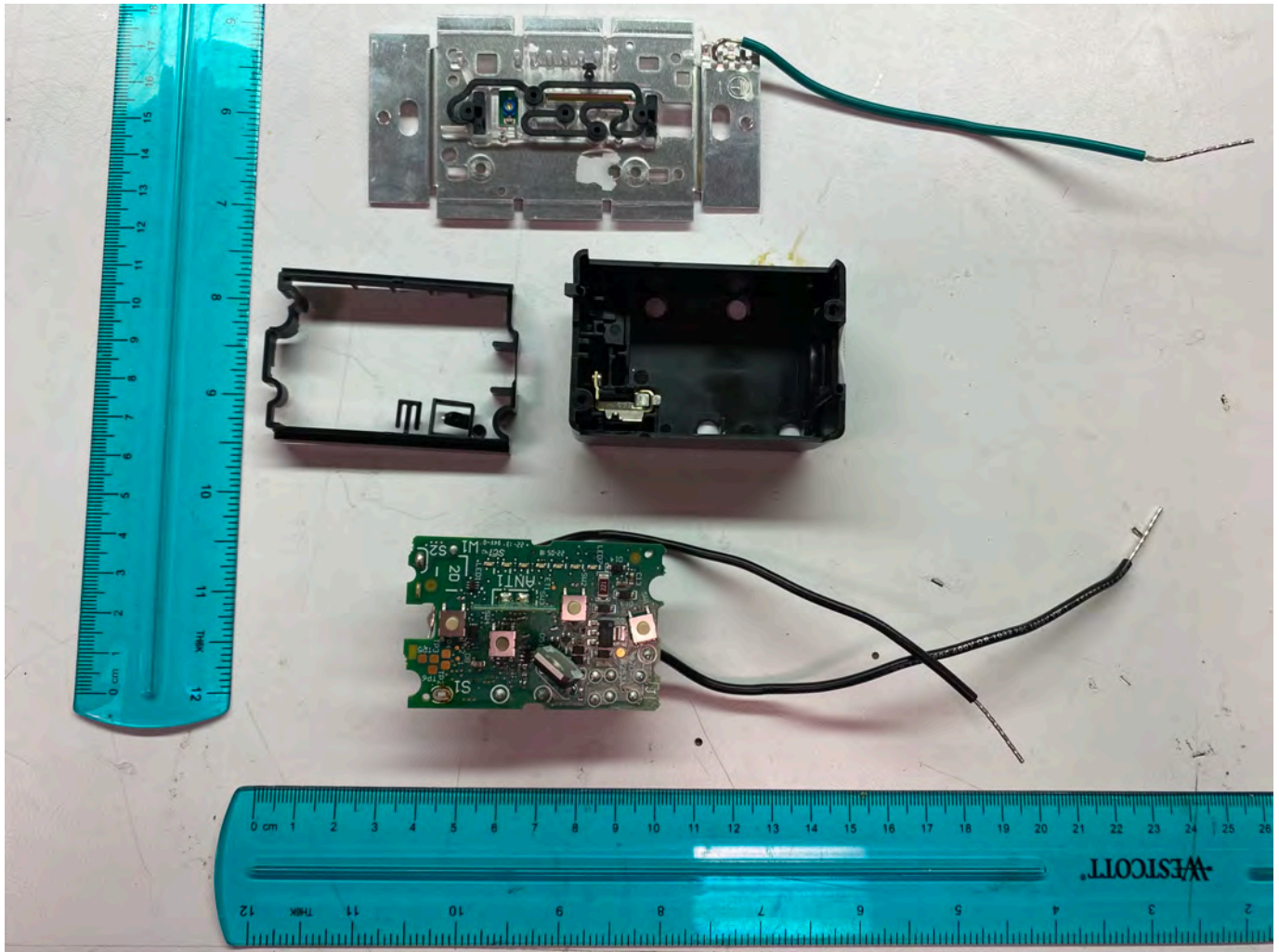
Top PCB
