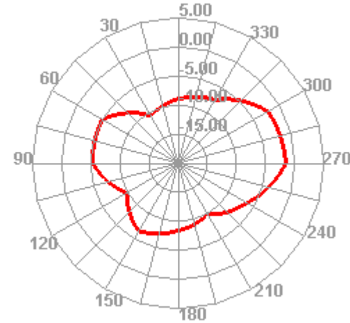
2450.000MHz Phi=45
