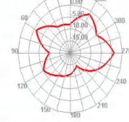
5350.000MHz E2
