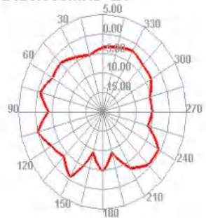
2425.000MHz E1
