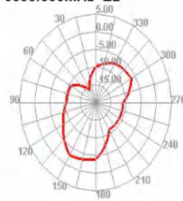
5350.000MHz E2
