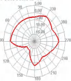
5750.000MHz E2
