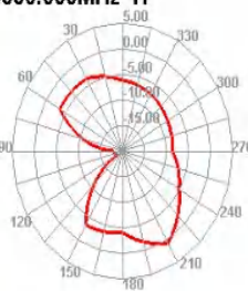
5550.000MHz H
