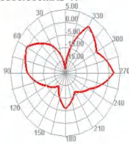
5550.000MHz H
