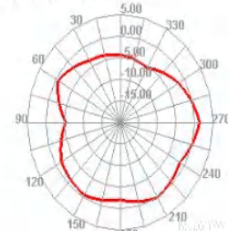
5250.000MHz E2
