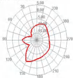
5150.000MHz E2
