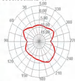
5350.000MHz E2
