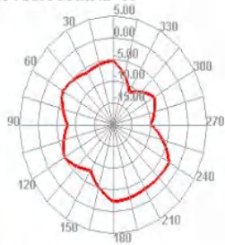
5150.000MHz E2
