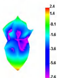
5150.000MHz E1
