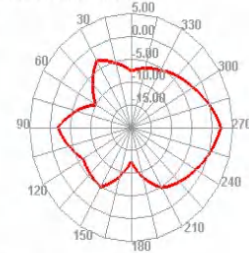
5150.000MHz E2
