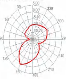
5550.000MHz E2
