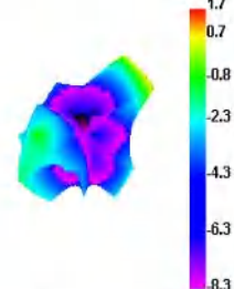
5350.000MHz E1
