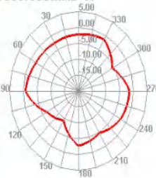
5850.000MHz H
