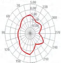
5250.000MHz E1
