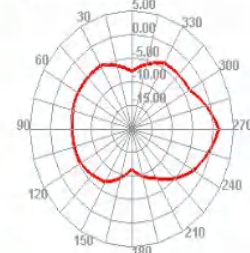
5250.000MHz H
