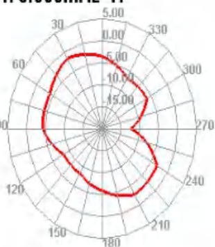
2475.000MHz E2
