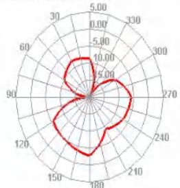
5550.000MHz E1
