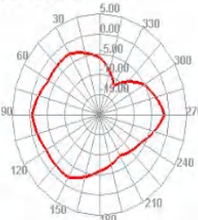
5850.000MHz E2
