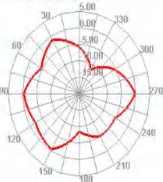
5750.000MHz E2
