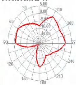
5650.000MHz E2
