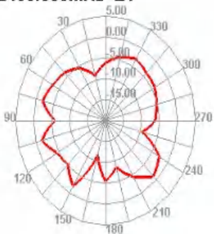
2400.000MHz E1
