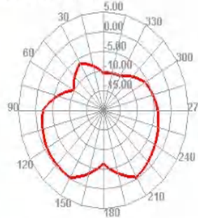
2450.000MHz E2
