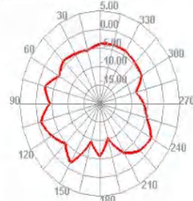
2450.000MHz E1
