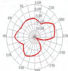
5850.000MHz E1
