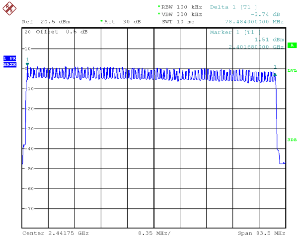
Modulation: \pi/4 DQPSK
