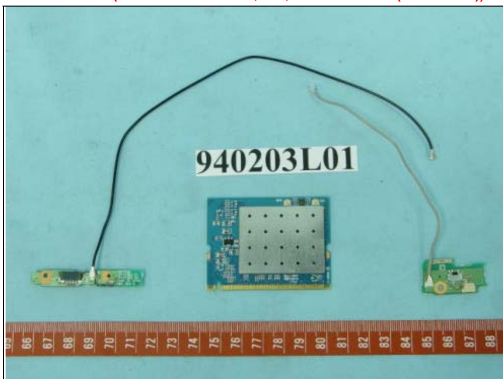
Antenna 12 (Brand: Yokowo Co., Ltd, P/N: YCE-5008(008L00197))
