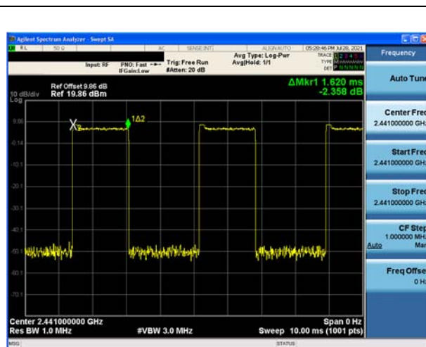
Modulation: \pi/4 DQPSK 2DH3 2441
