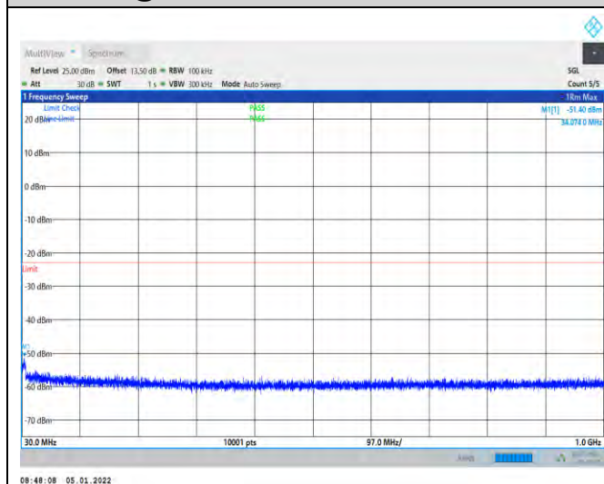
1-N66-PC3-15-40-L-4-DFT-QPSK-Edge_1RB_Left-1 @0-30-1000--51.40--23-PASS
