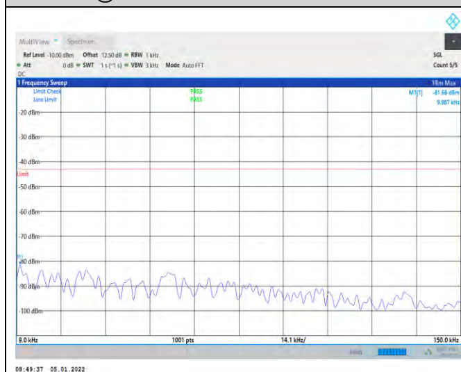
1-N66-PC3-15-40-M-4-DFT-QPSK-Edge_1RB_Left-1 @0-0.009-0.15--81.66--43-PASS
