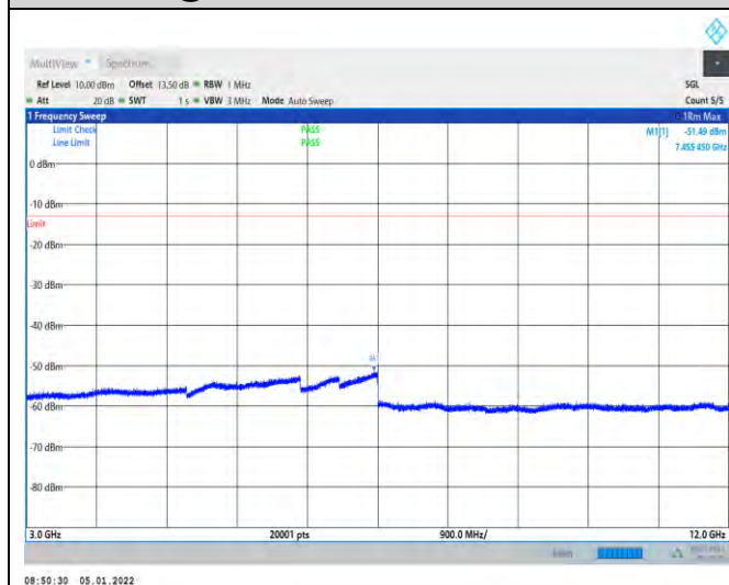
1-N66-PC3-15-40-M-4-DFT-QPSK-Edge_1RB_Left-1 @0-3000-12000--51.49--13-PASS
