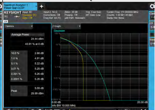
10MHz / 64QAM
