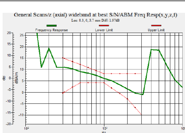
UMTS Band IV/1413CH(Battery 1#)
