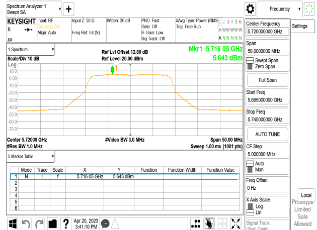
802.11n_20MHz_Chain1_5720MHz_UNII 3
