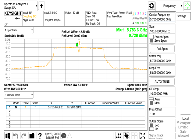
802.11n_40MHz_Chain0_5755MHz
