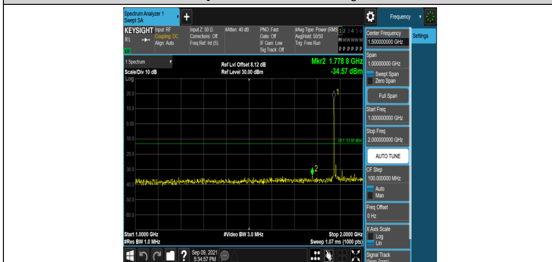
Band25-20MHz-QPSK-26365-1RB#0-Range4:1000~2000MHz
