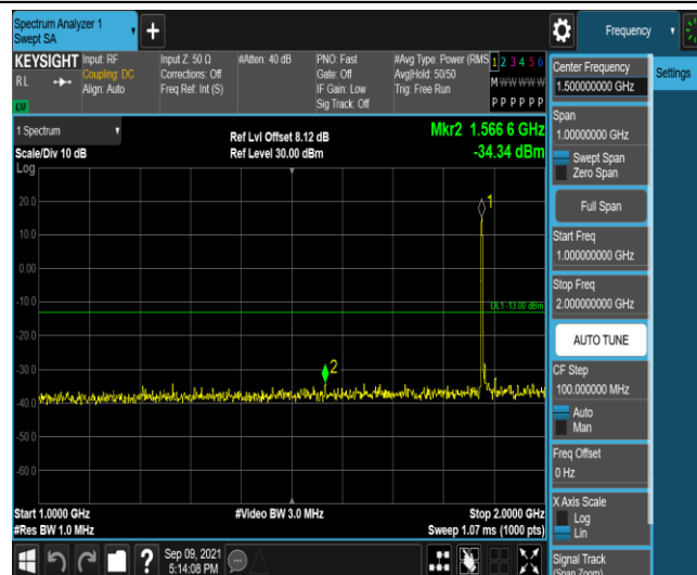
Band25-15MHz-QPSK-26365-1RB#0-Range4:1000~2000MHz
