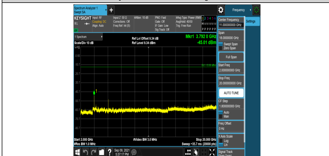
Band25-20MHz-QPSK-26590-1RB#0-Range5:2000~20000MHz
