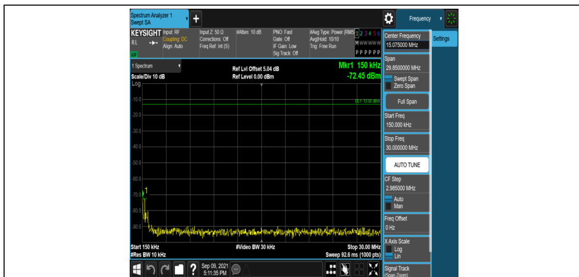
Band25-15MHz-QPSK-26115-1RB#0-Range2:0.15~30MHz
