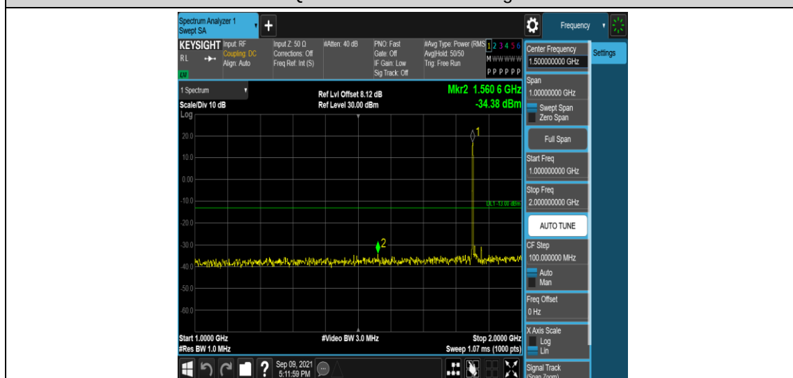
Band25-15MHz-QPSK-26115-1RB#0-Range4:1000~2000MHz
