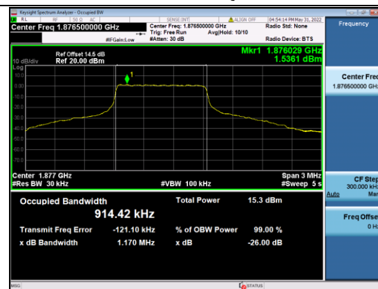
B25-15M-Mid CH-OBW-Q16
