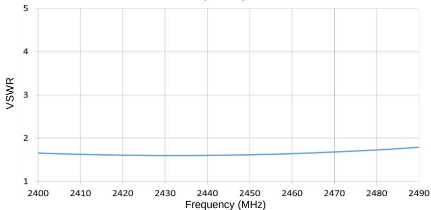
2.4 GHz VSWR
