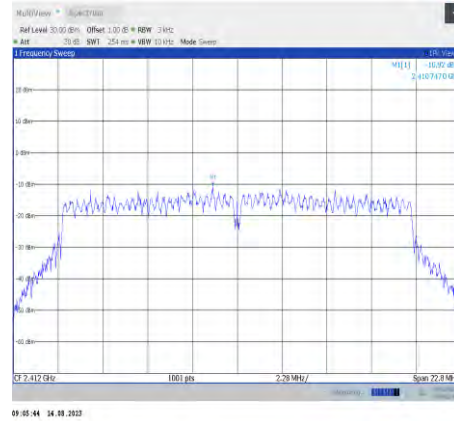
11n20MIMO-Ant8-2412
