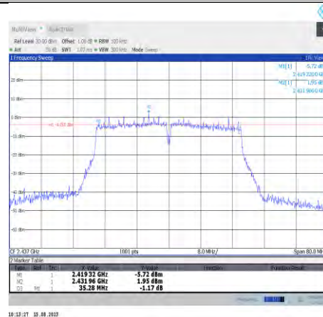
11n40MIMO-Ant8-2437
