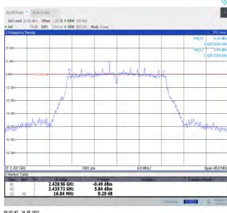
11n20MIMO-Ant10-2437
