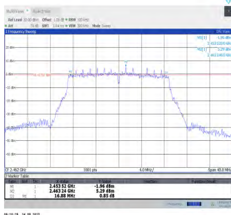
11n20MIMO-Ant10-2462
