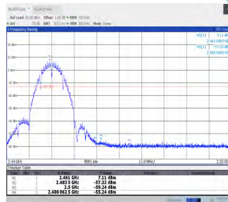
11b-CDD-Ant8-2462
