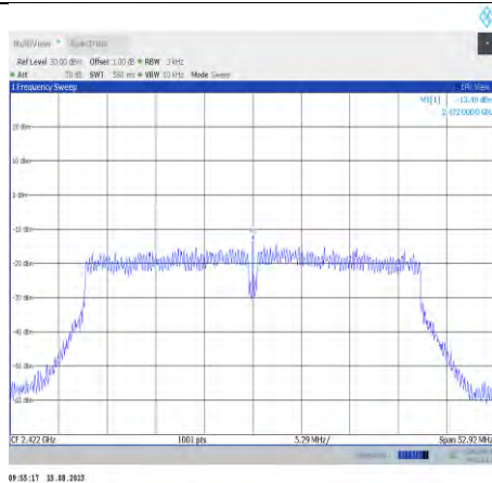
11n40MIMO-Ant10-2422
