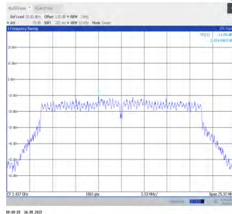
11n20MIMO-Ant8-2437
