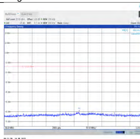
11n20MIMO-Ant10-2462-30~1000
