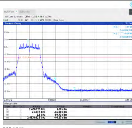
11n20MIMO-Ant8-2462
