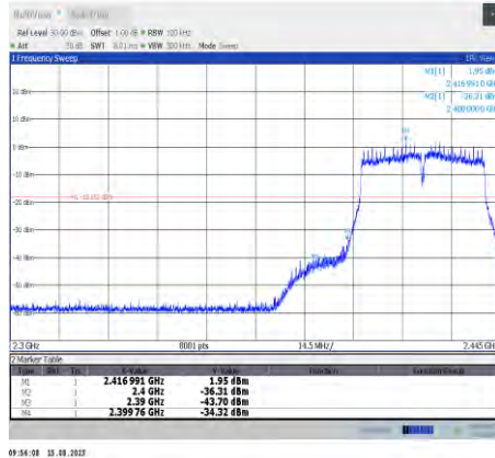
11n40MIMO-Ant10-2422
