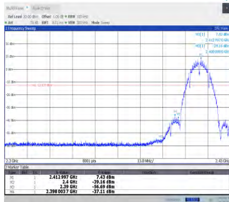
11b-CDD-Ant10-2412
