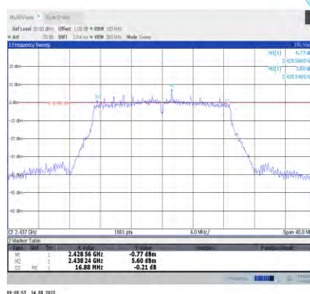
11n20MIMO-Ant8-2437
