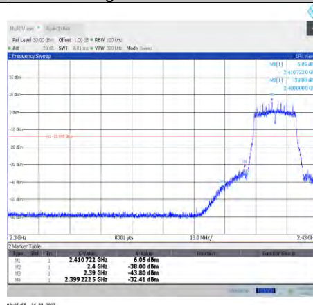
11n20MIMO-Ant8-2412
