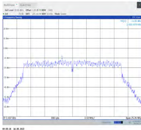
11n20MIMO-Ant10-2437
