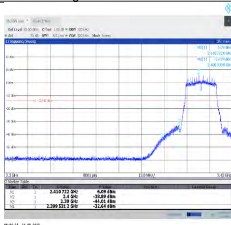
11n20MIMO-Ant10-2412
