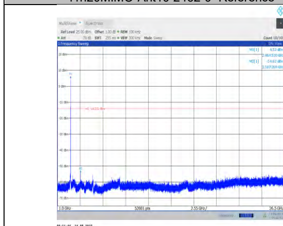
11n20MIMO-Ant10-2462-1000~26500
