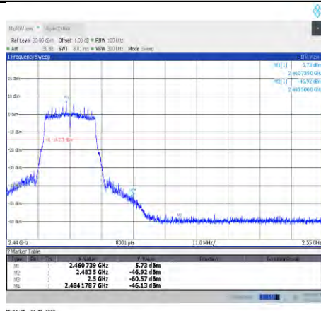
11n20MIMO-Ant10-2462
