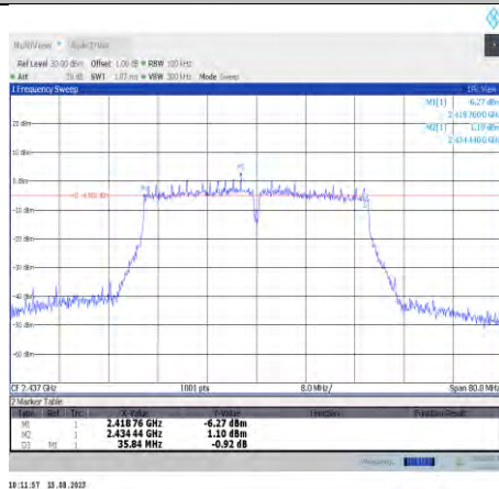
11n40MIMO-Ant10-2437
