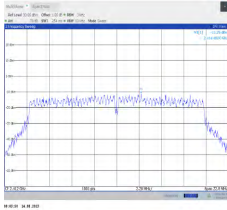
11n20MIMO-Ant10-2412
