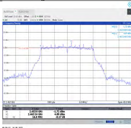
11g-CDD-Ant10-2462
