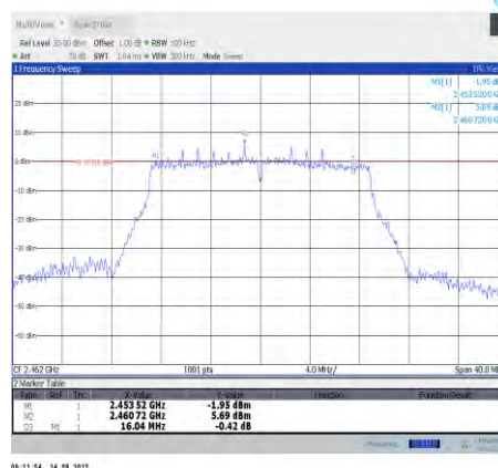
11n20MIMO-Ant8-2462
