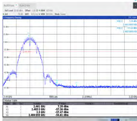
11b-CDD-Ant10-2462
