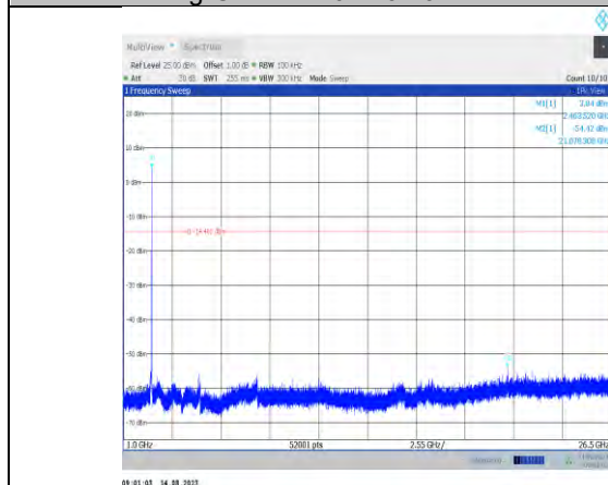
11g-CDD-Ant10-2462-1000~26500
