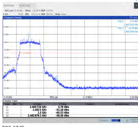
11g-CDD-Ant10-2462
