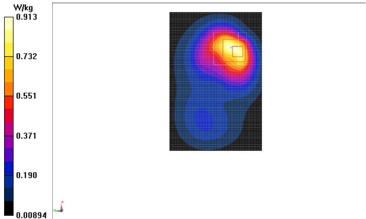
Fig.10 WCDMA1900
